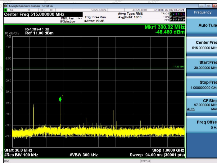
2.4G-Ant1-2474-30~1000-PASS
