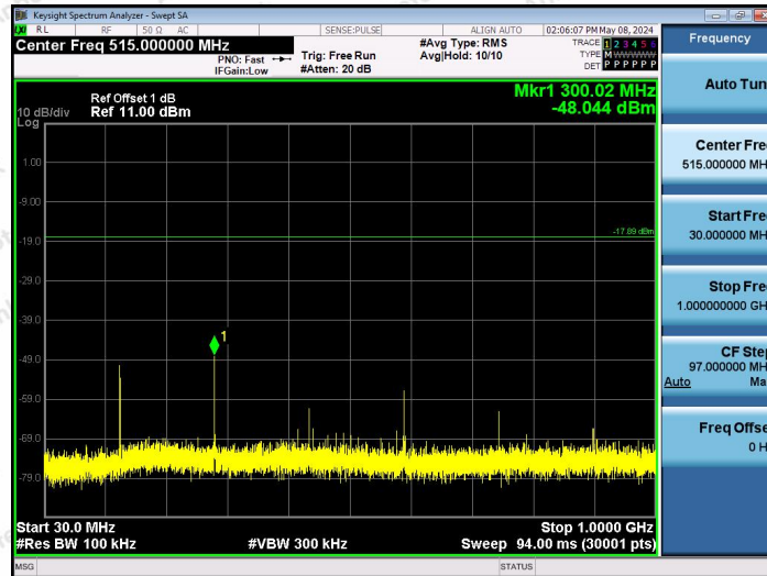
2.4G-Ant1-2408-30~1000-PASS
