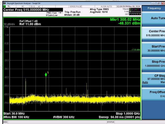
2.4G-Ant1-2440-30~1000-PASS
