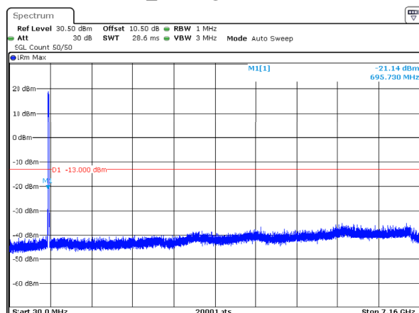
n12_15MHz_15kHz_706.5MHz_DFT-s-OFDM QPSK_RB75@0 -21.14dBm
