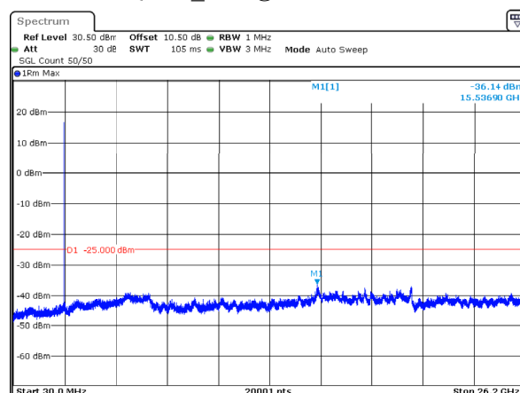
n38_5MHz_15kHz_2572.5MHz_DFT-s-OFDM QPSK_RB1@0 -36.14dBm
