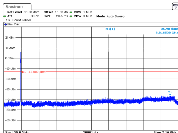
n12_15MHz_15kHz_708.5MHz_DFT-s-OFDM QPSK_RB1@0 -35.90dBm
