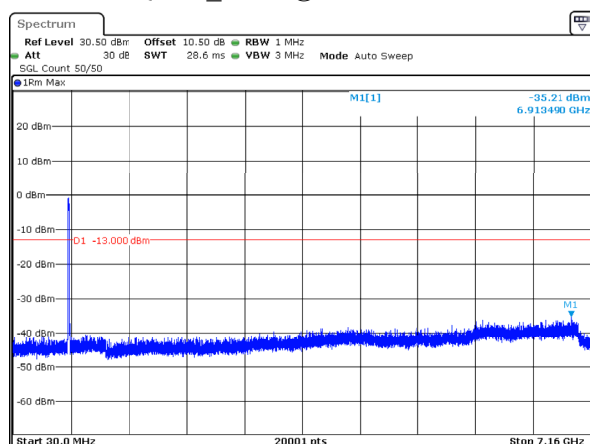
n12_15MHz_15kHz_707.5MHz_DFT-s-OFDM QPSK_RB75@0 -35.21dBm
