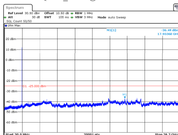
n38_5MHz_15kHz_2572.5MHz_DFT-s-OFDM QPSK_RB25@0 -36.49dBm
