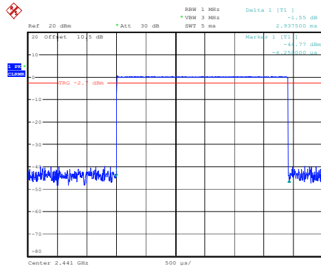
DH5_Hopping 2.938ms
