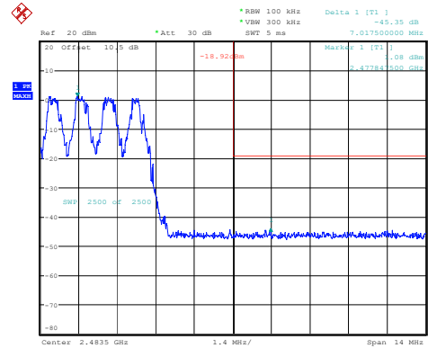
DH1_Hopping_Upper
