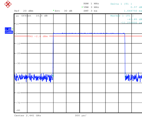
DH3_Hopping 1.669ms
