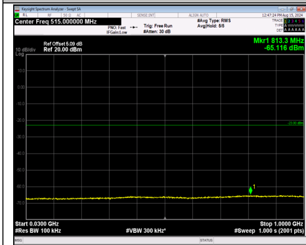
66-66-20MHz-20MHz-QPSK-QPSK-132072-132270-1RB #99-0RB#0-30~1000MHz-PASS
