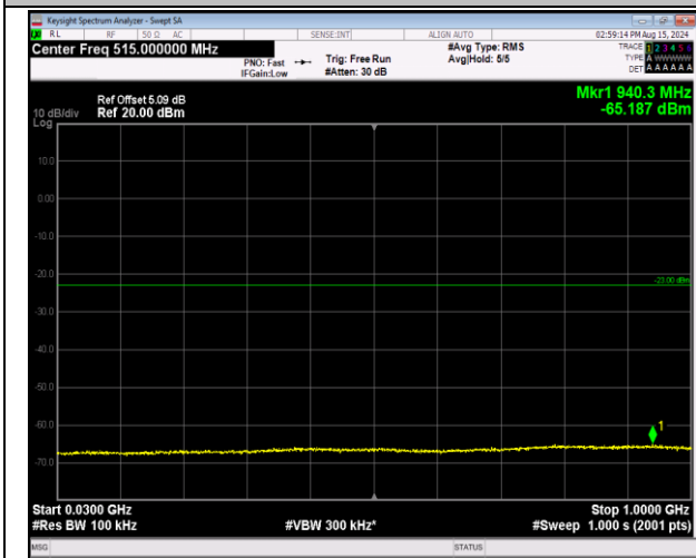
66-66-20MHz-20MHz-64QAM-64QAM-132072-132270-100RB#0-100RB#0-30~1000MHz-PASS
