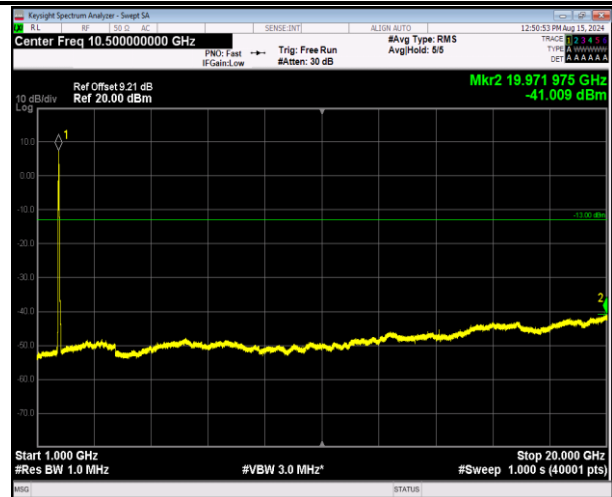
66-66-20MHz-20MHz-16QAM-16QAM-132072-132270-100 RB#0-100RB#0-1000~20000MHz-PASS
