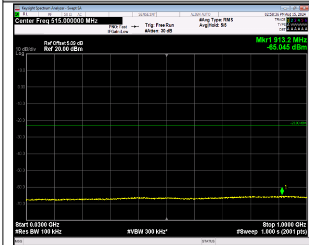
66-66-20MHz-20MHz-64QAM-64QAM-132072-132270-1 RB#0-1RB#99-30~1000MHz-PASS
