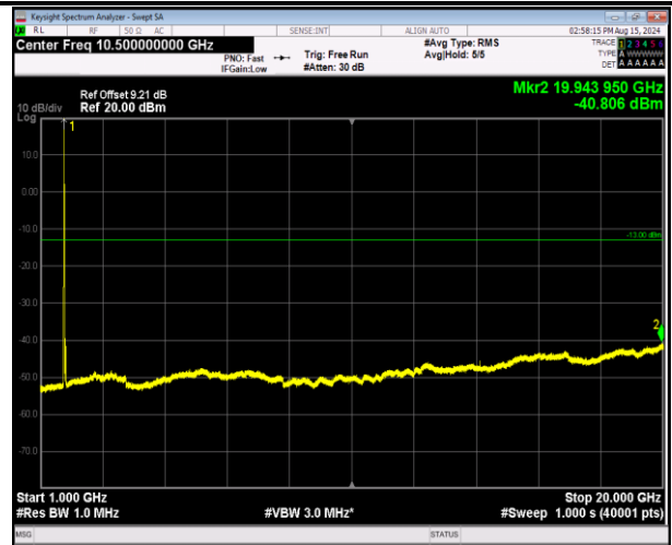
66-66-20MHz-20MHz-64QAM-64QAM-132072-132270-1RB #99-0RB#0-1000~20000MHz-PASS
