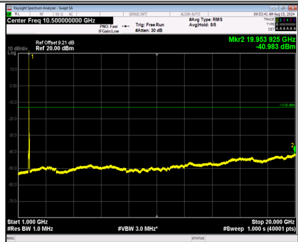
66-66-20MHz-5MHz-QPSK-QPSK-132397-132514-1RB#0- ORB#0-1000~20000MHz-PASS
