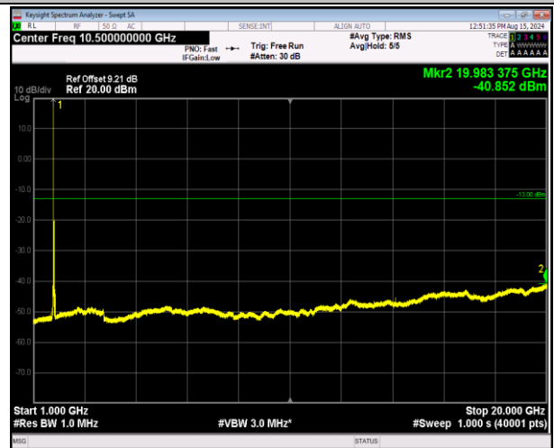
66-66-20MHz-20MHz-QPSK-QPSK-132323-132521-1RB#0-0RB#0-1000~20000MHz-PASS
