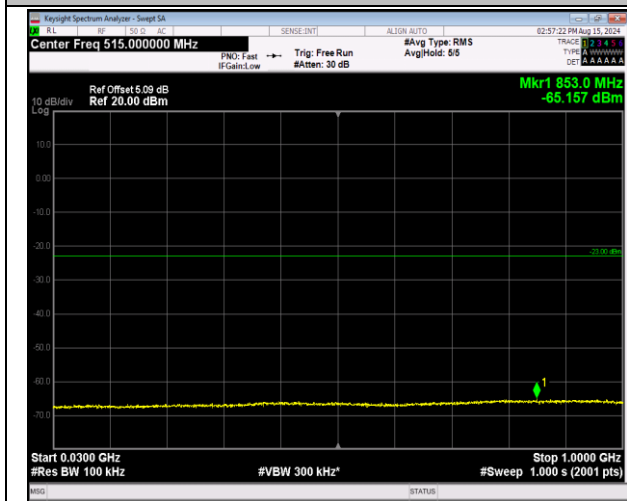
66-66-20MHz-20MHz-64QAM-64QAM-132072-132270-1 RB#0-0RB#0-30~1000MHz-PASS
