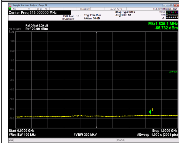
66-66-20MHz-5MHz-64QAM-64QAM-132072-132189-10 ORB#0-25RB#0-30~1000MHz-PASS
