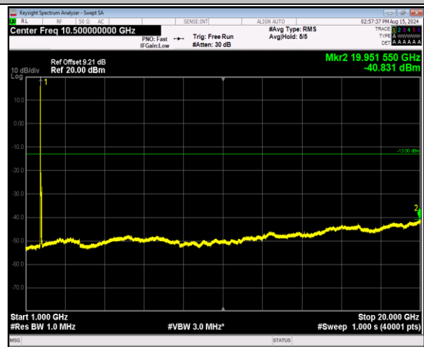
66-66-20MHz-20MHz-64QAM-64QAM-132072-132270-1RB #0-0RB#0-1000~20000MHz-PASS
