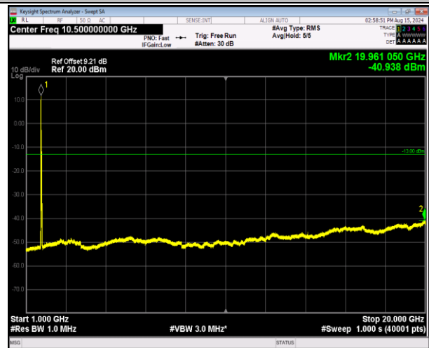
66-66-20MHz-20MHz-64QAM-64QAM-132072-132270-1RB #0-1RB#99-1000~20000MHz-PASS
