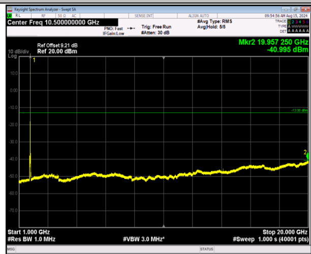
66-66-20MHz-5MHz-QPSK-QPSK-132397-132514-1RB#99 -0RB#0-1000~20000MHz-PASS
