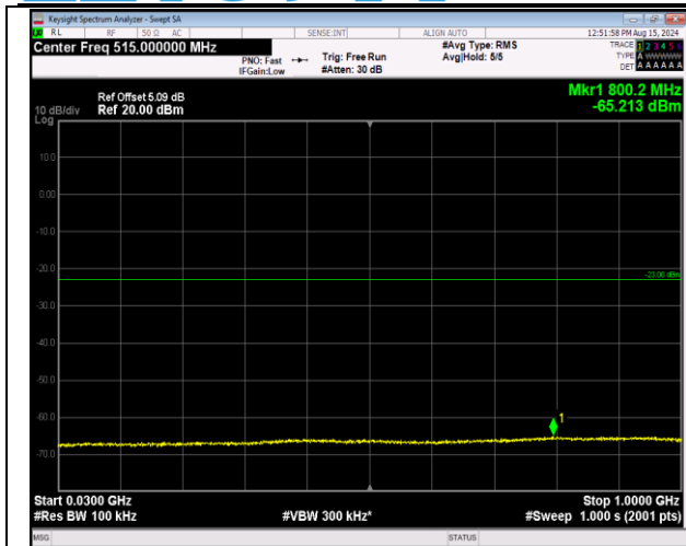
66-66-20MHz-20MHz-16QAM-16QAM-132323-132521-1 RB#0-ORB#0-30~1000MHz-PASS
