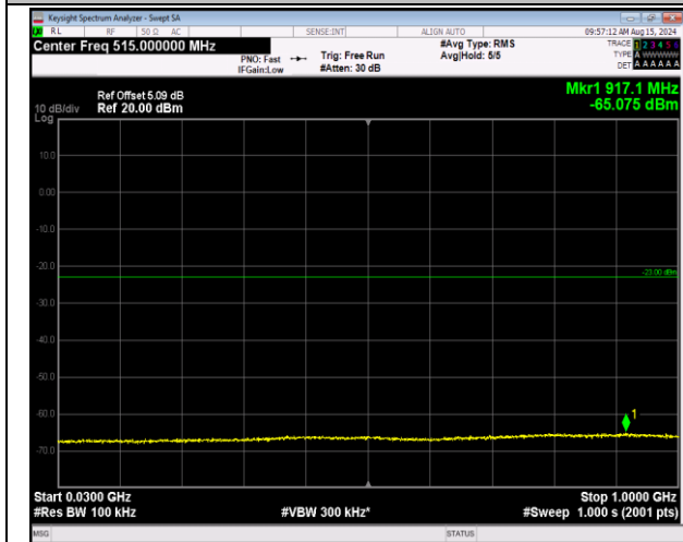
66-66-20MHz-5MHz-QPSK-QPSK-132397-132514-100R B#0-25RB#0-30~1000MHz-PASS
