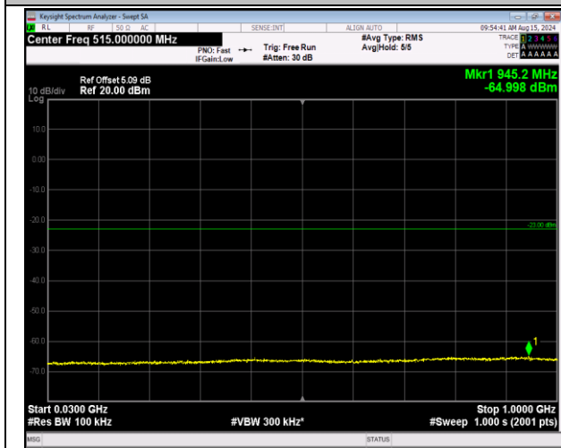
66-66-20MHz-5MHz-QPSK-QPSK-132397-132514-1RB# 99-0RB#0-30~1000MHz-PASS
