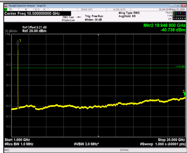
66-66-20MHz-5MHz-64QAM-64QAM-132072-132189-100R B#0-25RB#0-1000~20000MHz-PASS
