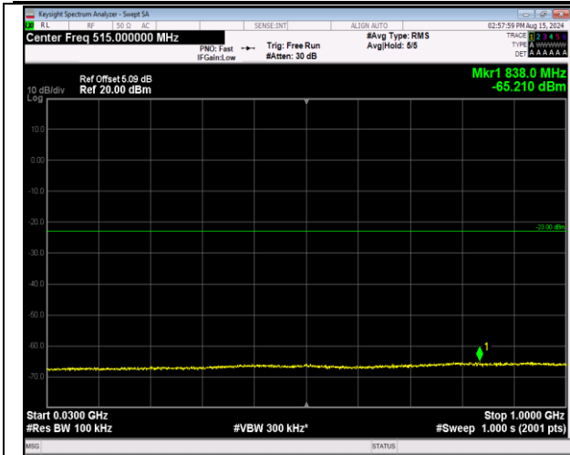
66-66-20MHz-20MHz-64QAM-64QAM-132072-132270-1RB RB#99-0RB#0-30~1000MHz-PASS
