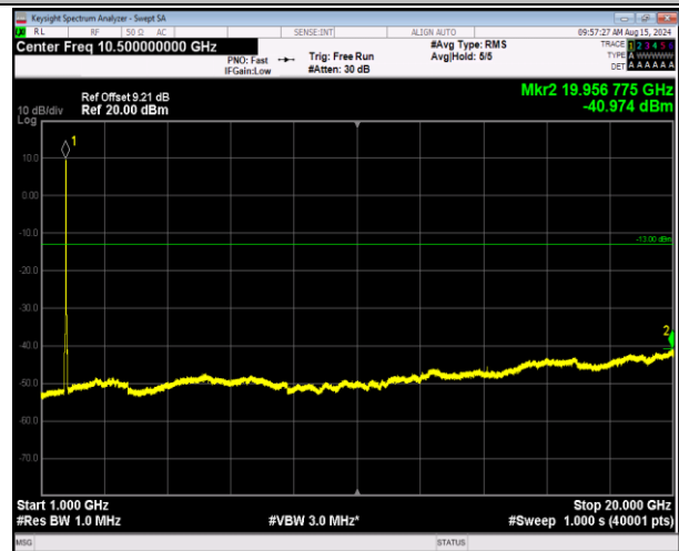
66-66-20MHz-5MHz-QPSK-QPSK-132397-132514-100RB# 0-25RB#0-1000~20000MHz-PASS
