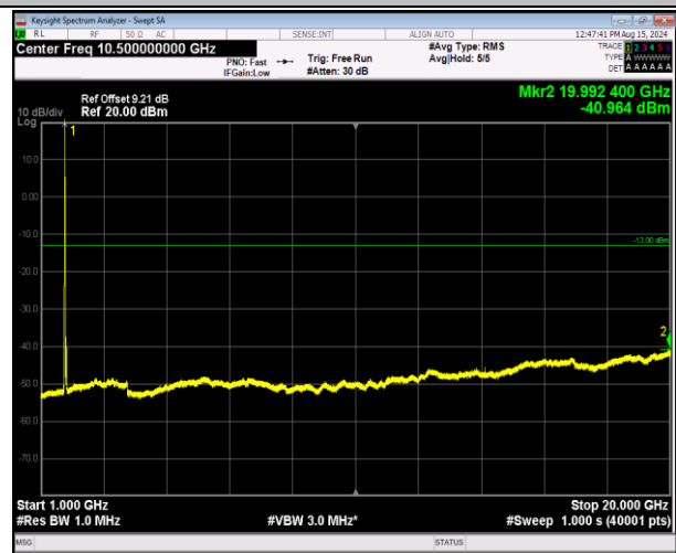
66-66-20MHz-20MHz-QPSK-QPSK-132072-132270-1RB#9 9-0RB#0-1000~20000MHz-PASS
