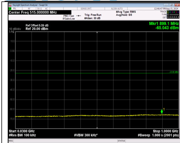
66-66-20MHz-20MHz-16QAM-16QAM-132072-132270-1 RB#0-ORB#0-30~1000MHz-PASS
