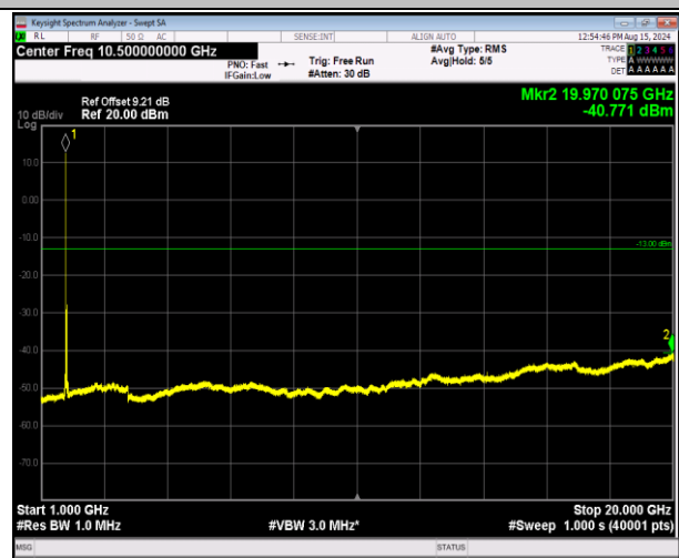
66-66-20MHz-20MHz-16QAM-16QAM-132323-132521-1RB #0-1RB#99-1000~20000MHz-PASS
