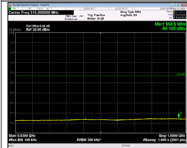
66-66-20MHz-20MHz-QPSK-QPSK-132323-132521-1RB#0-0RB#0-30~1000MHz-PASS
