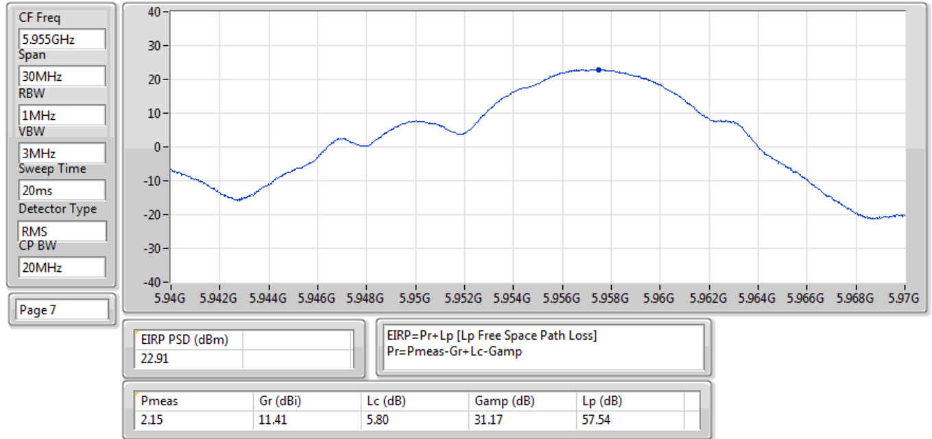
EIRP PSD;Band:6.2G;11a;BWch:20MHz;Nss:1,(6D);Nant:4;Ch:5955MHz;TX
