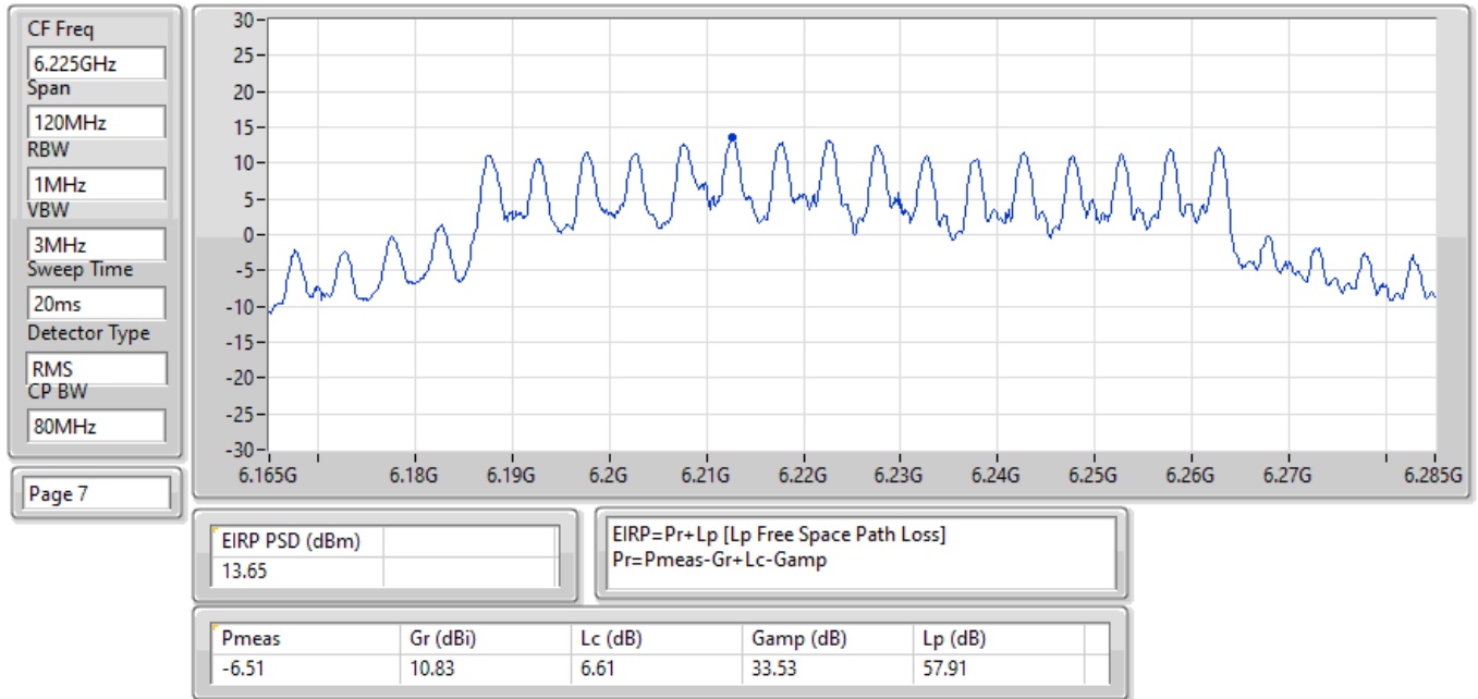
EIRP PSD;Band:6.2G;ax80;BWch:80MHz;Nss:1,(M0);Nant:4;Ch:6225MHz;TX
