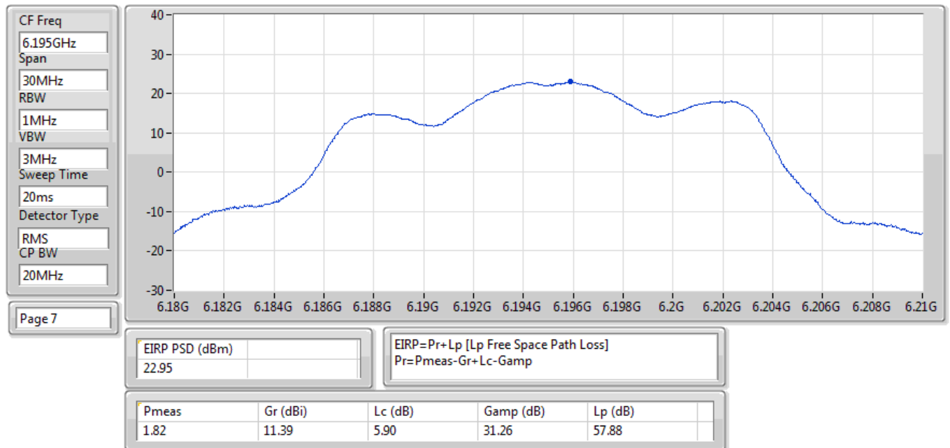
EIRP PSD;Band:6.2G;11a;BWch:20MHz;Nss:1,(6D);Nant:4;Ch:6195MHz;TX
