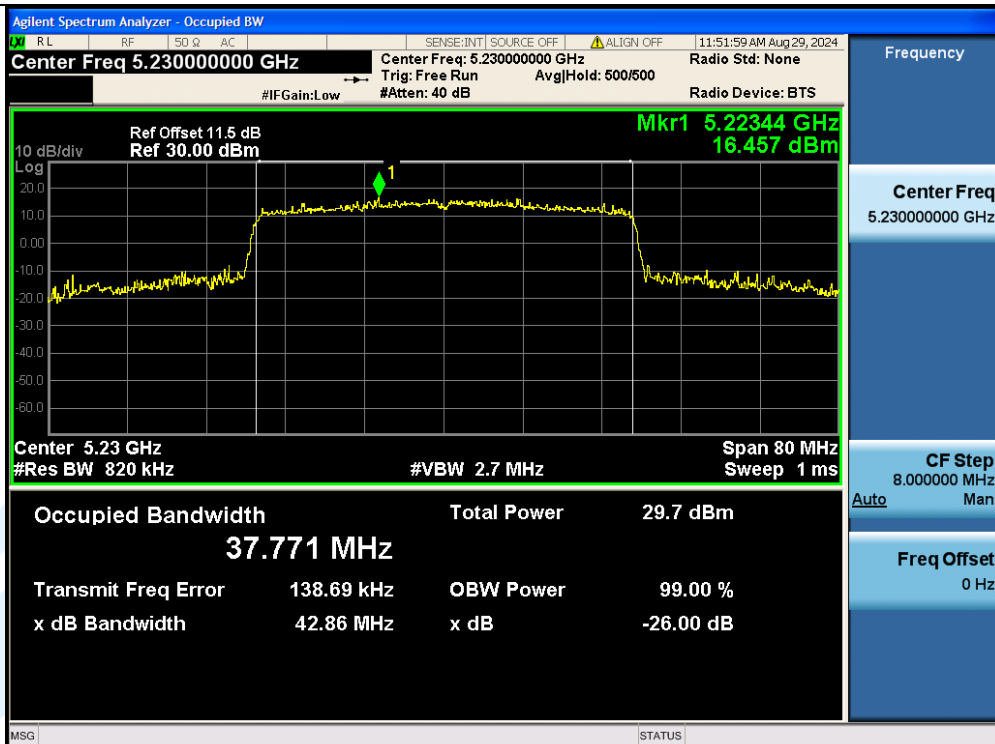
11AX40MIMO-Ant3-5230
