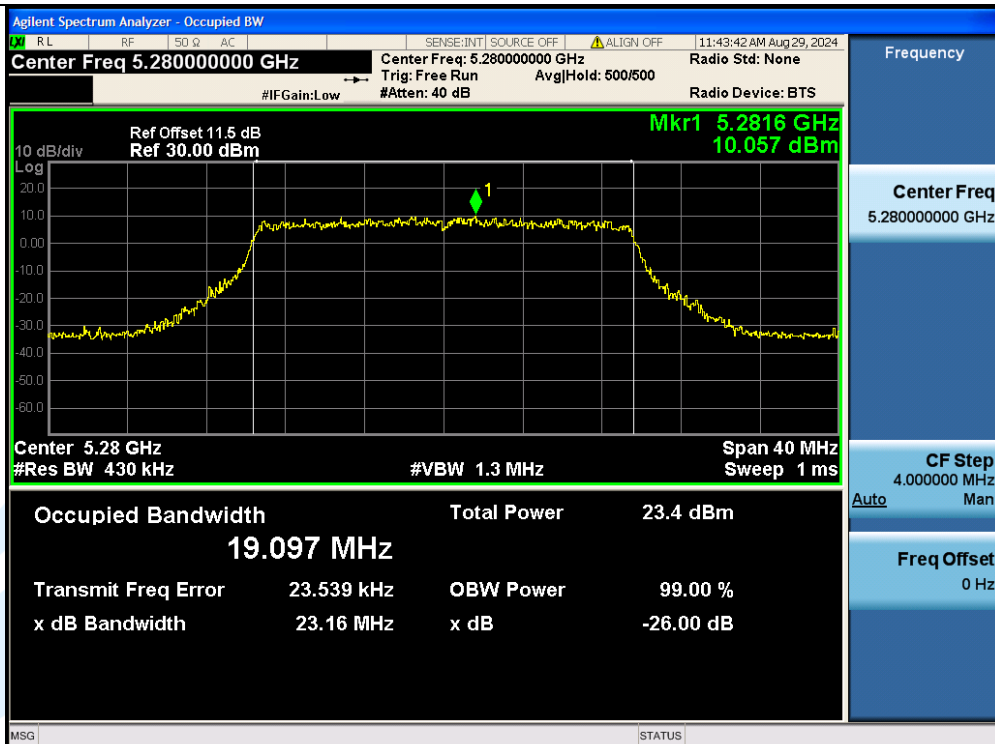
11AX20MIMO-Ant3-5280
