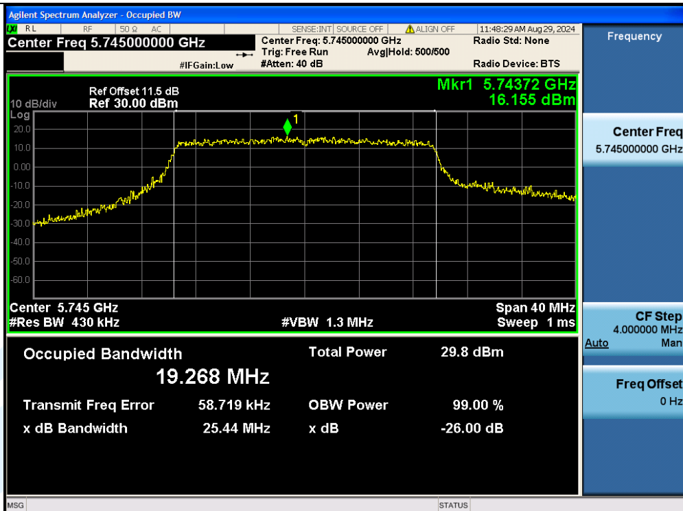
11AX20MIMO-Ant3-5745
