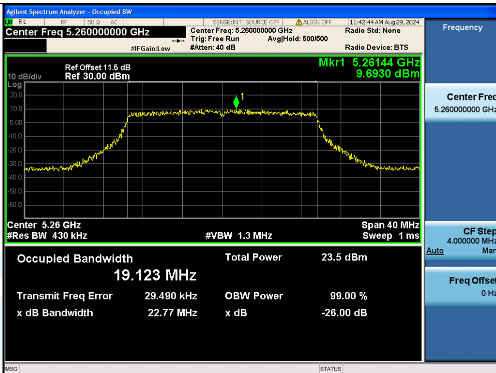
11AX20MIMO-Ant3-5260
