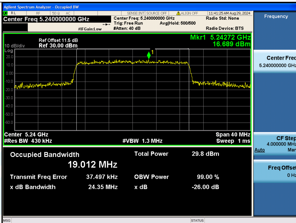
11AX20MIMO-Ant3-5240
