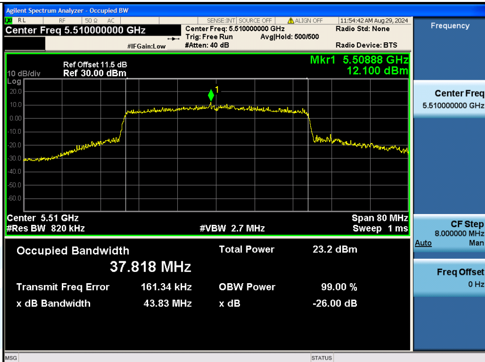
11AX40MIMO-Ant3-5510
