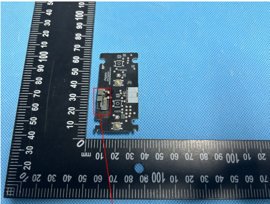
BT/Zigbee/Thread Ant.
