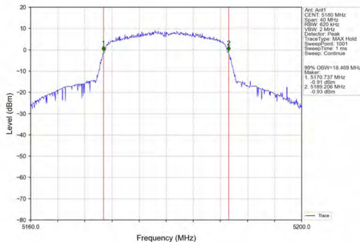
802.11n(HT20)_LCH_5180MHz_Ant1_NTNV
