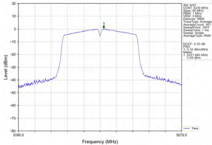
802.11n(HT40)_HCH_5230MHz_Ant1_NTNV
