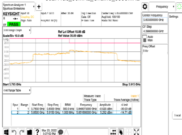
802.11ac_80MHz_Chain0_5855MHz
