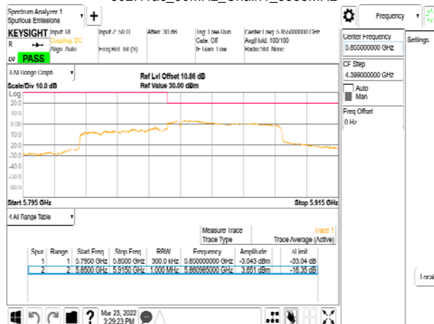
802.11ac_80MHz_Chain1_5855MHz
