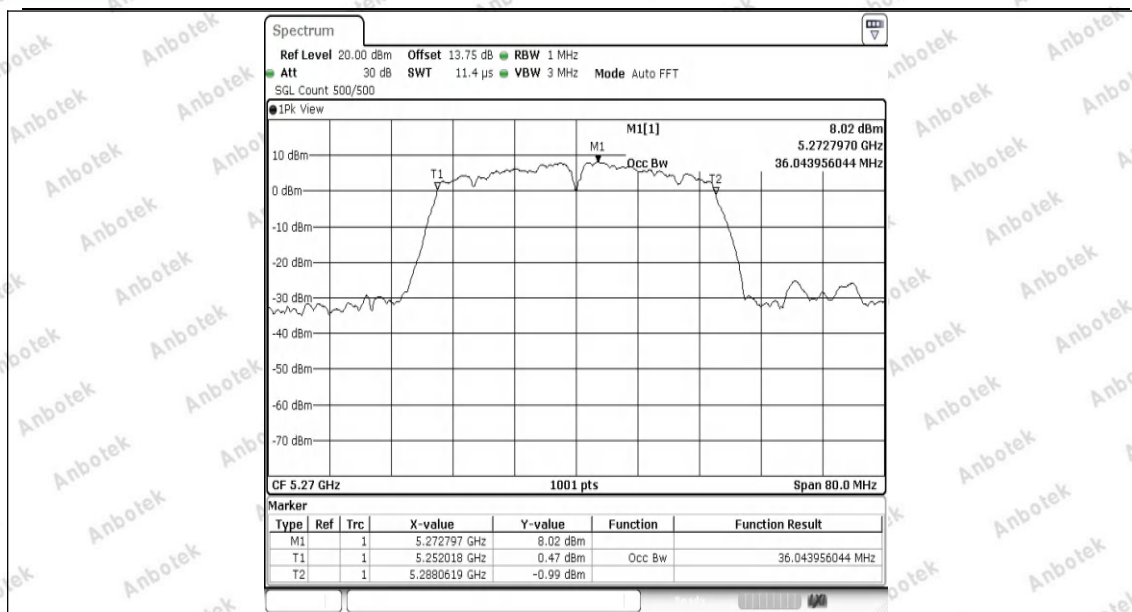
11N40SISO-Ant1-5270
