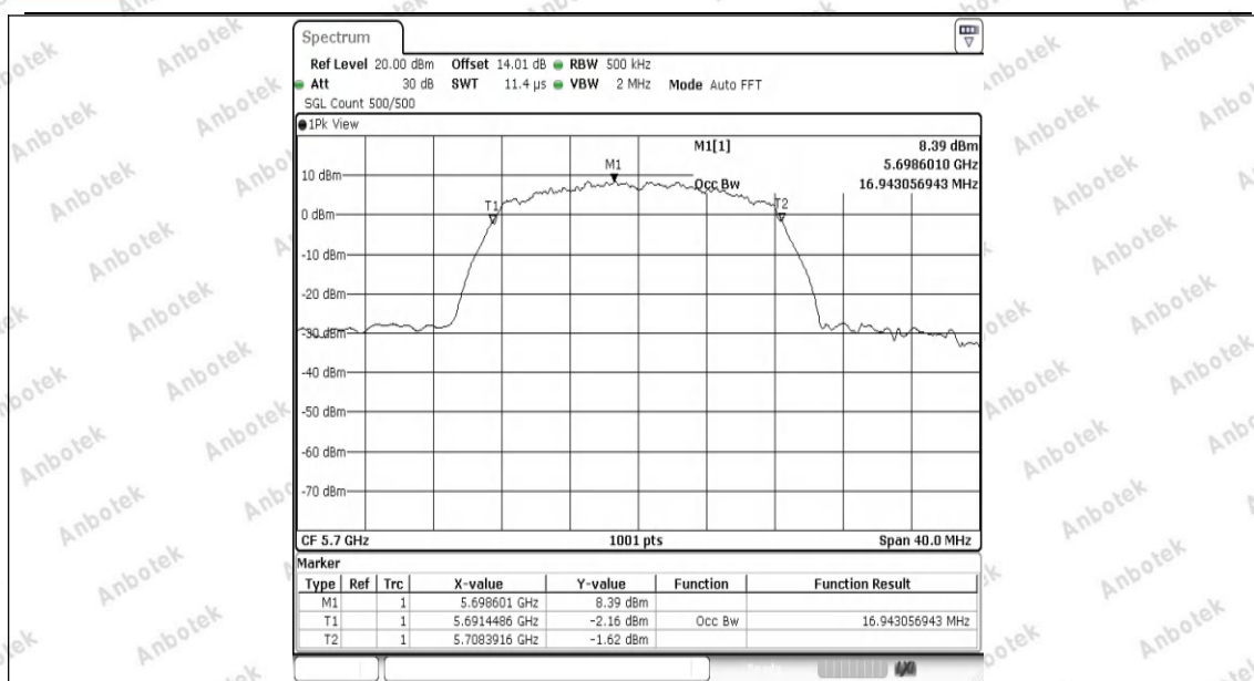
11A-Ant1-5700
