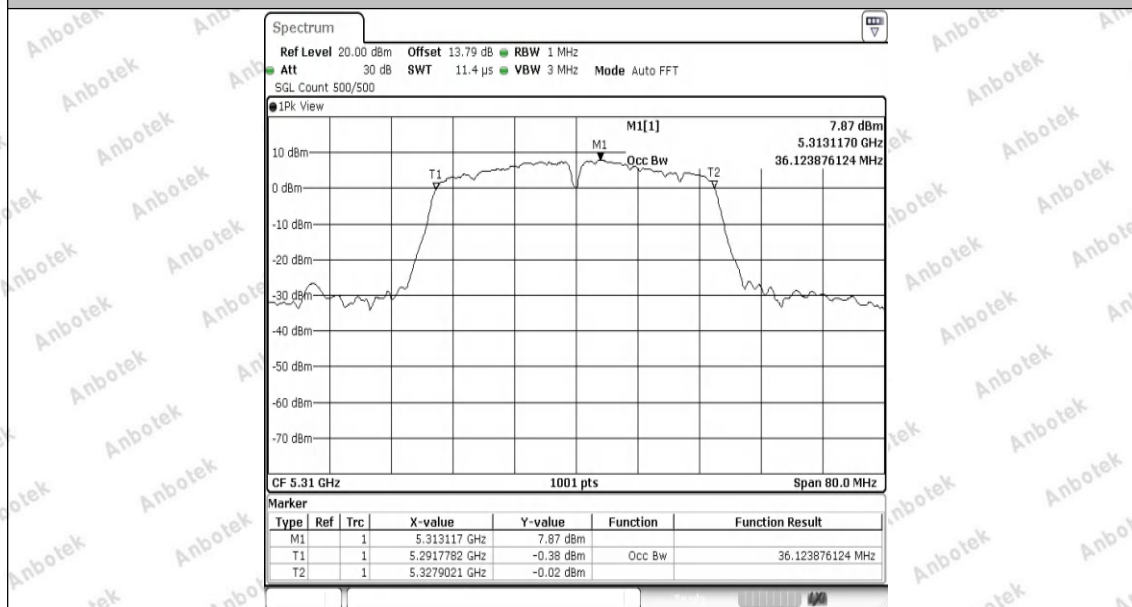
11N40SISO-Ant1-5310
