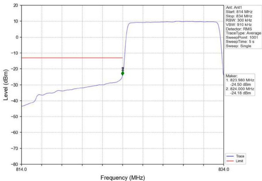
Band5_10MHz_QPSK_LCH_829MHz_RB_50_0_NTNV
