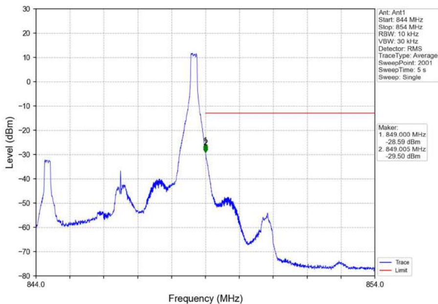
Band5_5MHz_QPSK_HCH_846.5MHz_RB_1_24_NTNV
