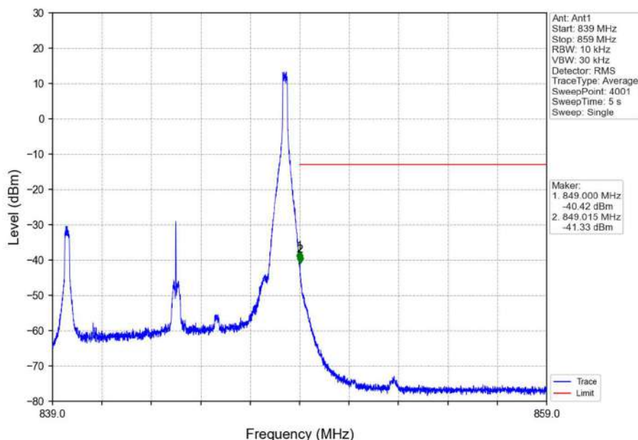
Band5_10MHz_QPSK_HCH_844MHz_RB_1_49_NTNV
