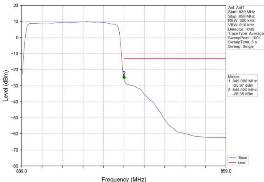
Band5_10MHz_QPSK_HCH_844MHz_RB_50_0_NTNV
