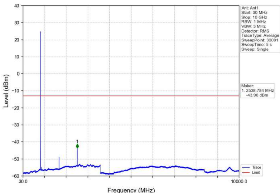
Band5_3MHz_QPSK_HCH_847.5MHz_RB_1_0_NTNV
