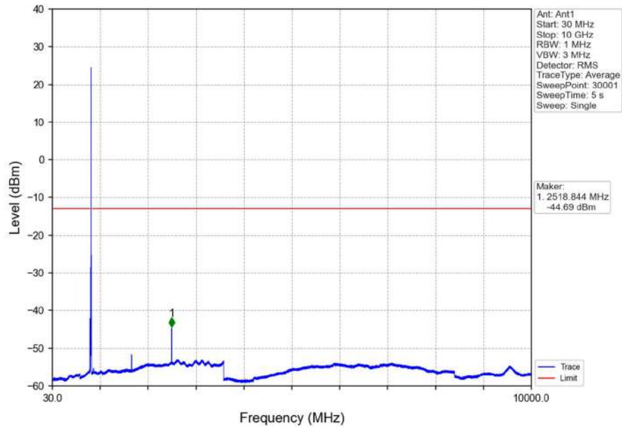
Band5_10MHz_QPSK_HCH_844MHz_RB_1_0_NTNV
