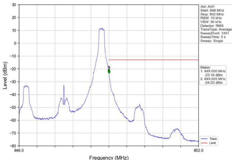
Band5_3MHz_QPSK_HCH_847.5MHz_RB_1_14_NTNV
