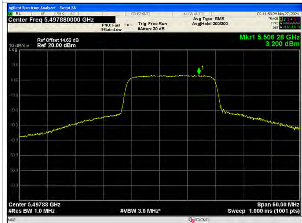
PSD NVNT ax40 242@61 5510MHz Ant1
