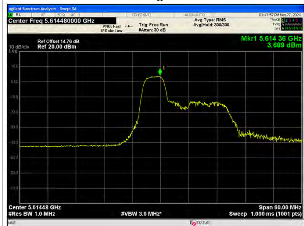
PSD NVNT ax40 52@37 5630MHz Ant1
