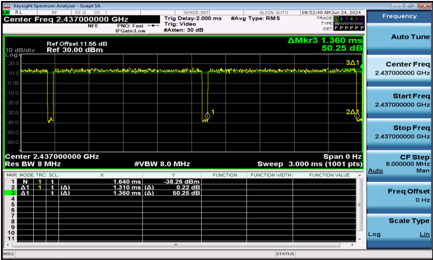
NTNV-11N20MIMO-Ant2-2437
