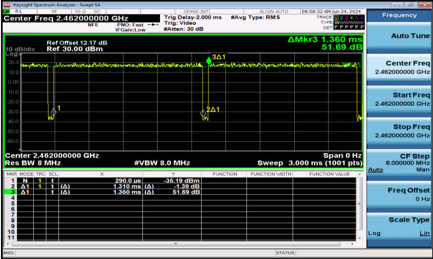
NTNV-11N20MIMO-Ant1-2462
