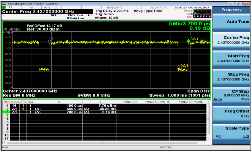
NTNV-11N40MIMO-Ant1-2437
