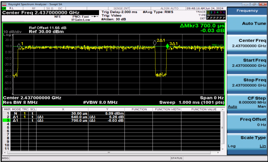
NTNV-11N40MIMO-Ant2-2437
