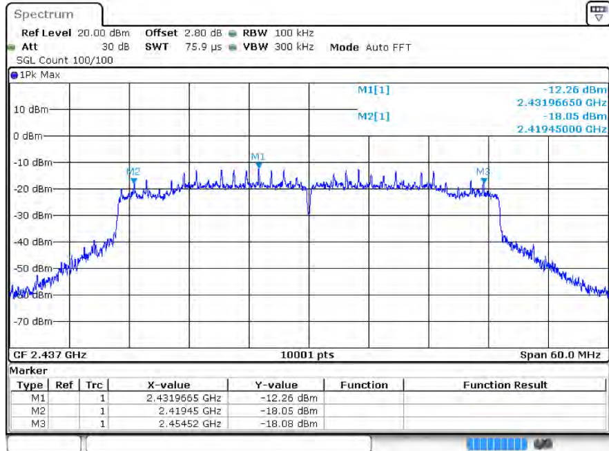
ax40 2437MHz Ant1
