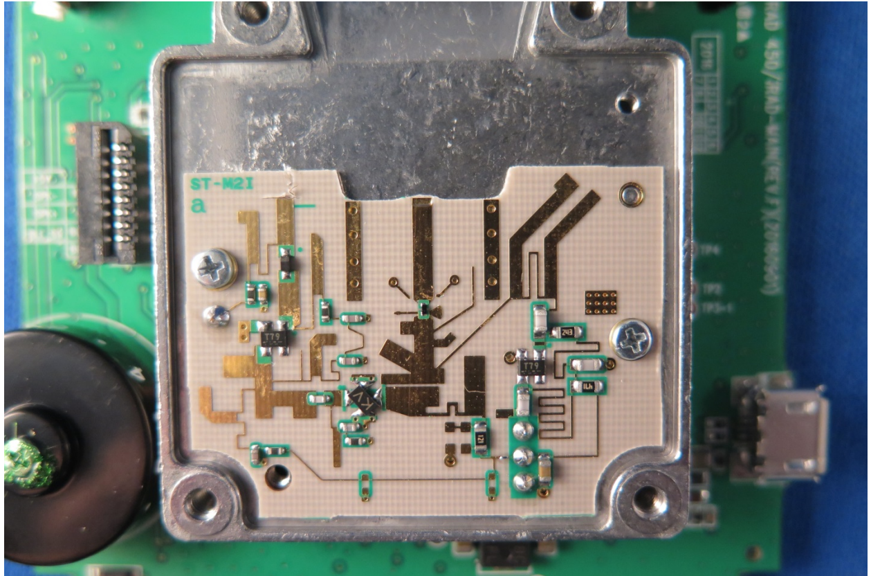
LNA PCB
