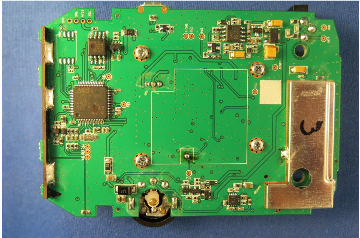
BOTTOM PCB
