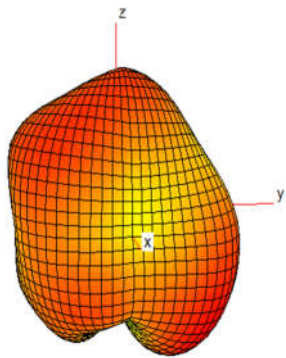
2450MHZ
