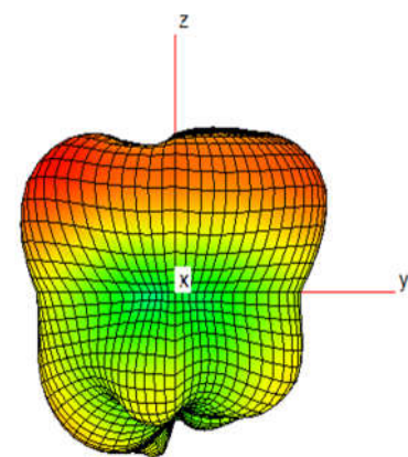
6500MHZ
