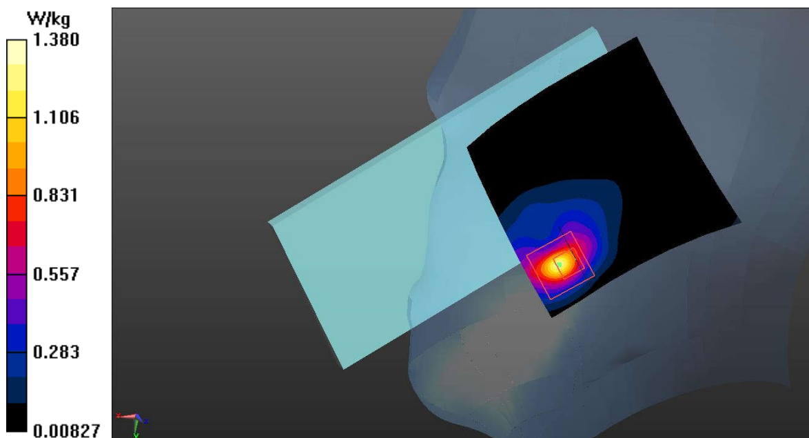
Fig.67 NR n66 Head
