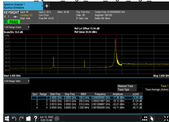
N78(60M)_DFT-s-OFDM QPSK Edge 1RB Right High CH
