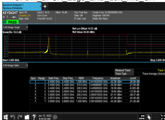
N78(100M)_DFT-s-OFDM BPSK Edge 1RB Left Mid CH
