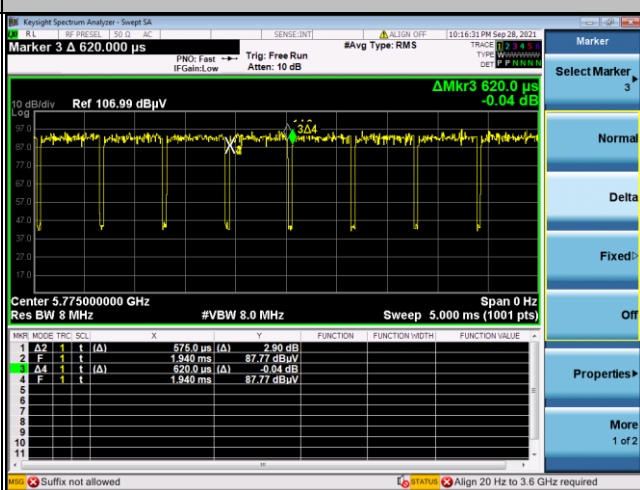
5GHz 802.11ax HE80 484 RU
