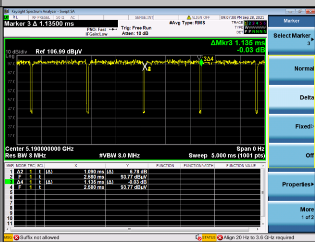
5GHz 802.11ax HE40 242 RU
