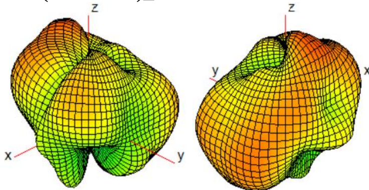
Ant7(WiFi0/BT)_6500
