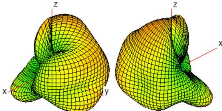
Ant8(WiFi1/BT)_6500
