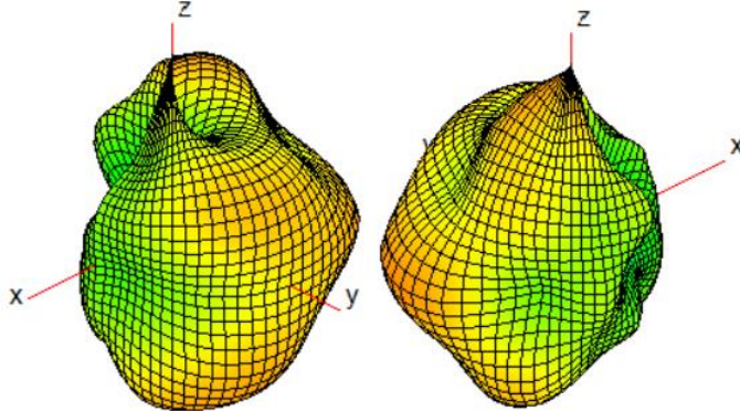
Ant8(WiFi1/BT)_5300
