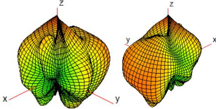
Ant8(WiFi1/BT)_2450
