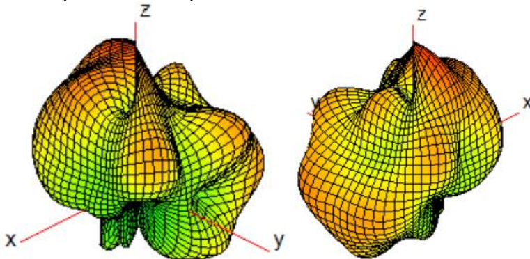
Ant7(WiFi0/BT)_6750
