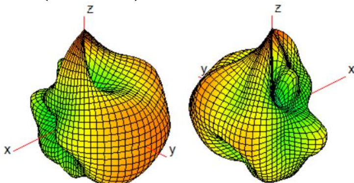
Ant8(WiFi1/BT)_6500
