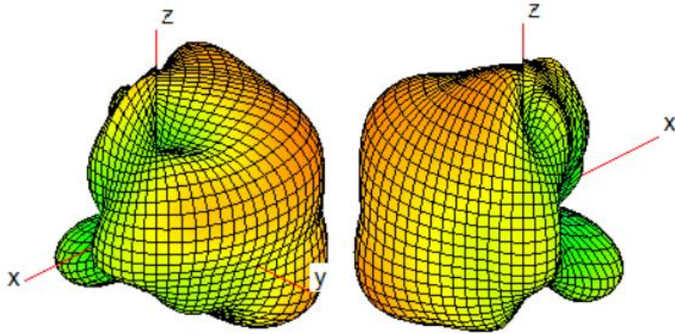
Ant8(WiFi1/BT)_7000
