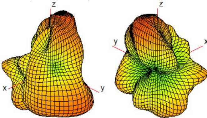
Ant8(WiFi1/BT)_5200
