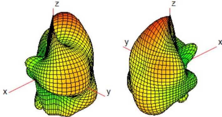
Ant8(WiFi1/BT)_5800
