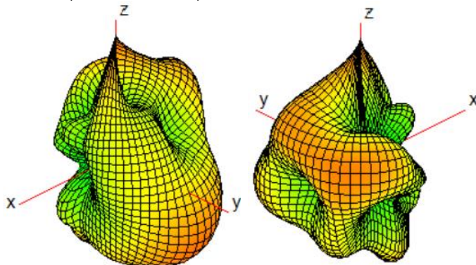
Ant8(WiFi1/BT)_6200
