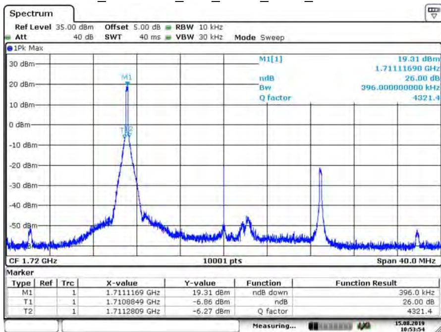
B66_CH132072_20M_QPSK_1RB0_26dB BW
