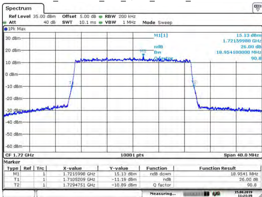
B66_CH132072_20M_QPSK_100RB0_26dB BW
