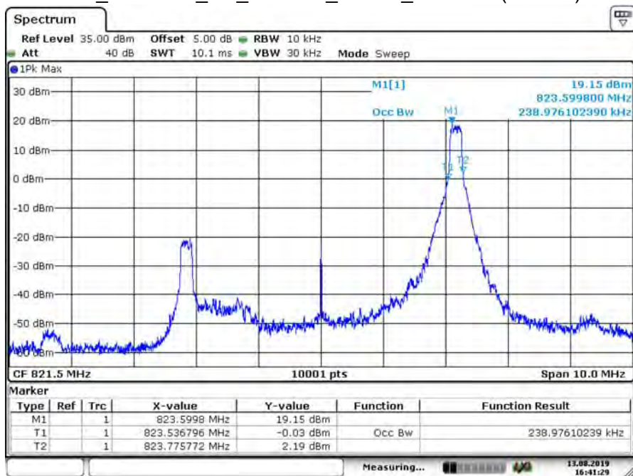
B26_CH26765_5M_16-QAM_1RB24_99% BW (Part 90)
