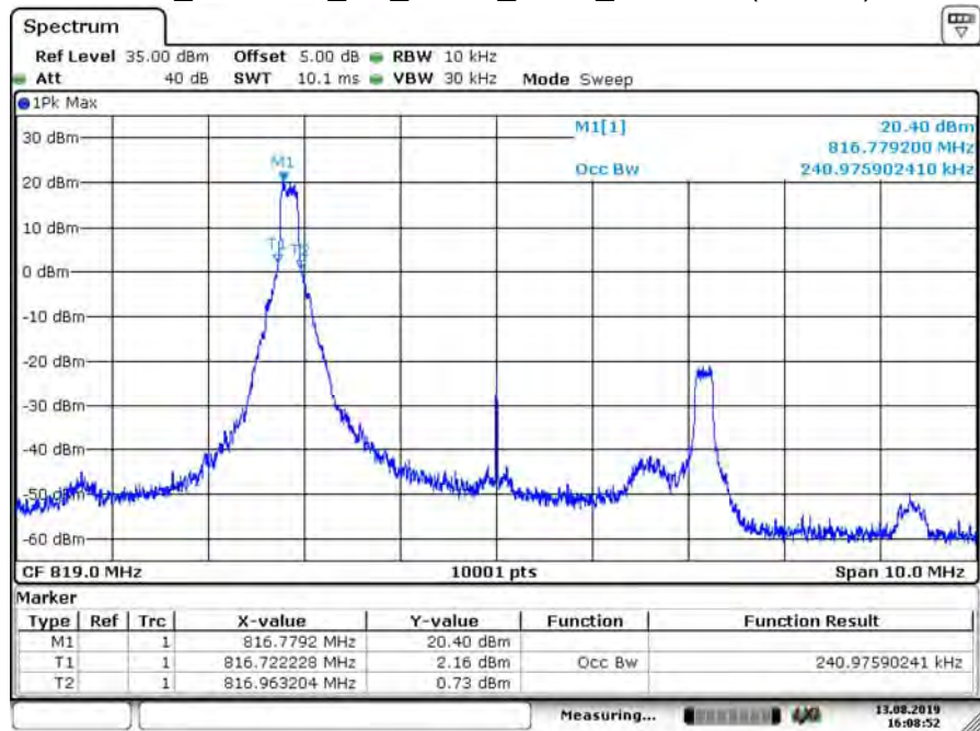
B26_CH26740_5M_QPSK_1RB0_99% BW (Part 90)
