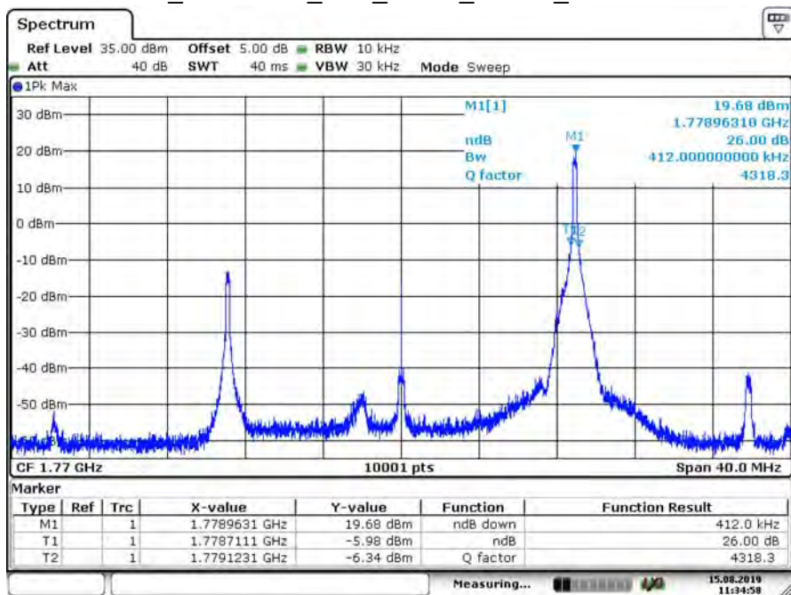
B66_CH132572_20M_QPSK_1RB99_26dB BW
