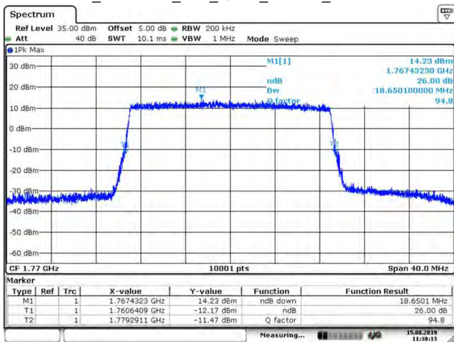
B66_CH132572_20M_QPSK_100RB0_26dB BW
