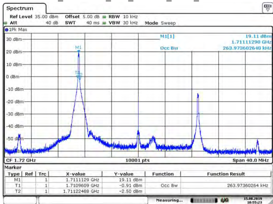
B66_CH132072_20M_16-QAM_1RB0_99% BW
