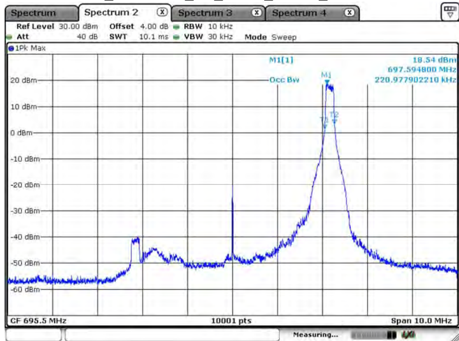
B71_CH133447_5M_QPSK_1RB24_99% BW
