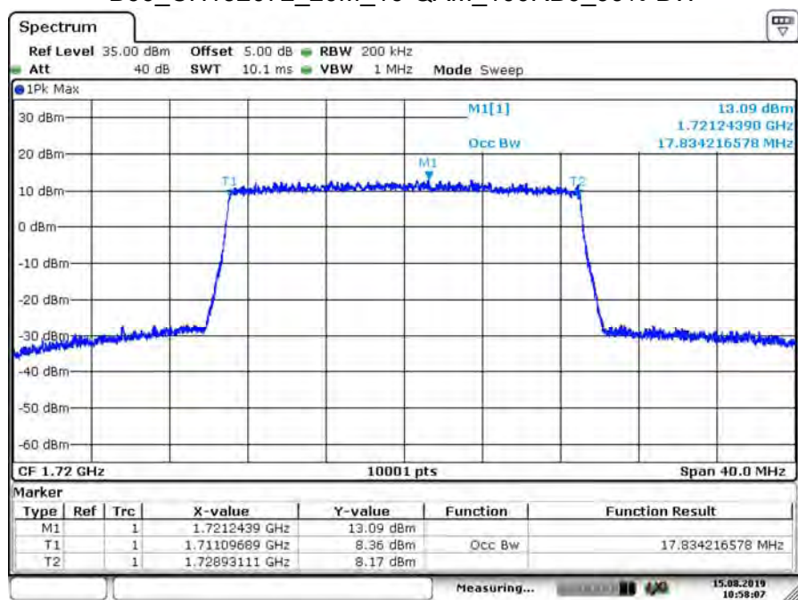
B66_CH132072_20M_16-QAM_100RB0_99% BW
