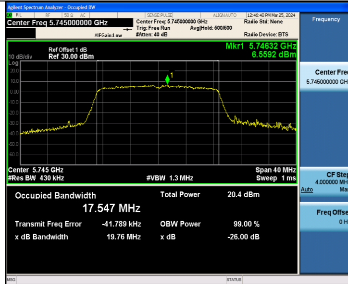
11N20MIMO_Ant2_5745
