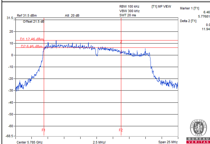
802.11a / Chain2 : CH 157
