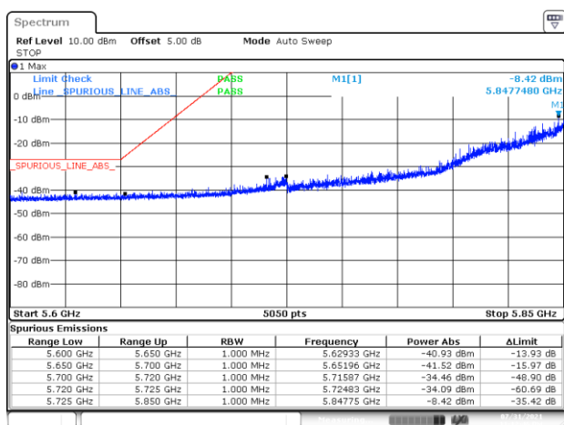
BE-NR-LOW, SISO-A, 802.11ax40-MCS0, Ch175
