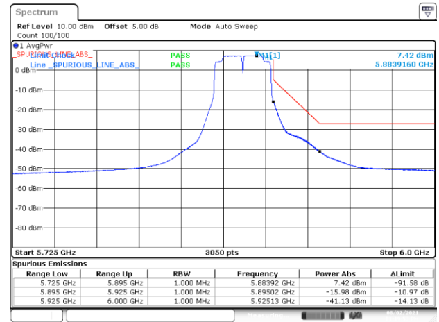
BE-NR-HIGH, MIMO-B, 802.11n40-HT0, Ch175
