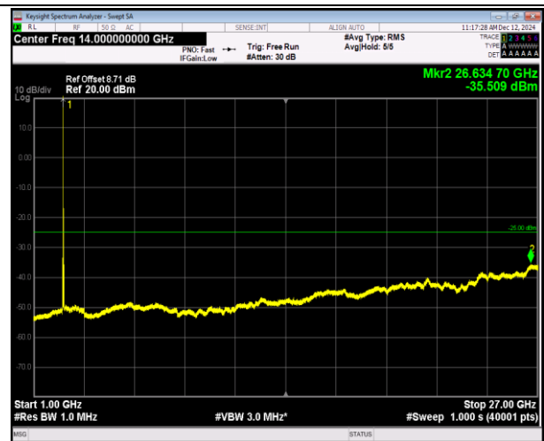
7-7-10MHz-20MHz-QPSK-QPSK-21006-21150-1RB#0-0RB #0-1000~27000MHz-PASS
