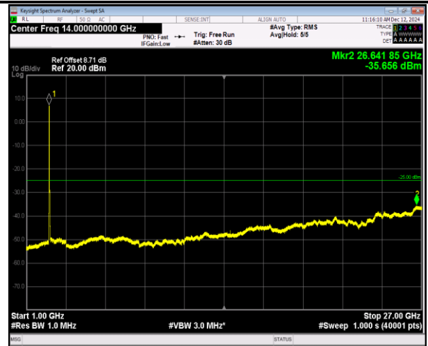
7-7-10MHz-20MHz-QPSK-QPSK-20805-20949-50RB#0-10 0RB#0-1000~27000MHz-PASS
