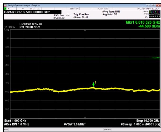
5-5-10MHz-10MHz-QPSK-QPSK-20501-20600-50RB#0-50 RB#0-1000~10000MHz-PASS
