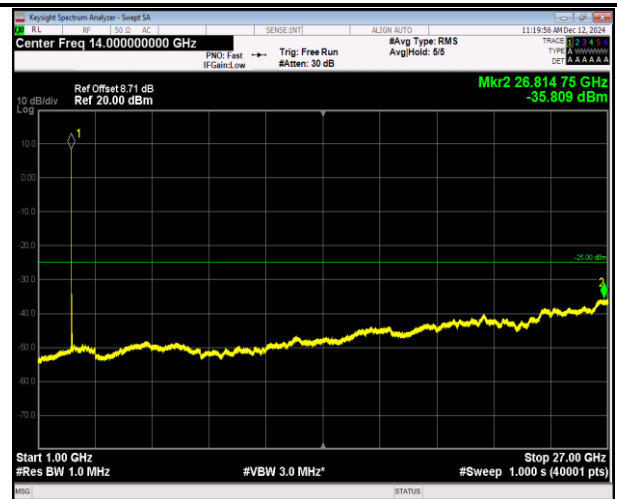
7-7-10MHz-20MHz-QPSK-QPSK-21006-21150-1RB#0-1RB #99-1000~27000MHz-PASS
