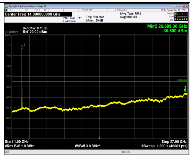
7-7-10MHz-20MHz-QPSK-QPSK-20805-20949-1RB#0-1RB #99-1000~27000MHz-PASS
