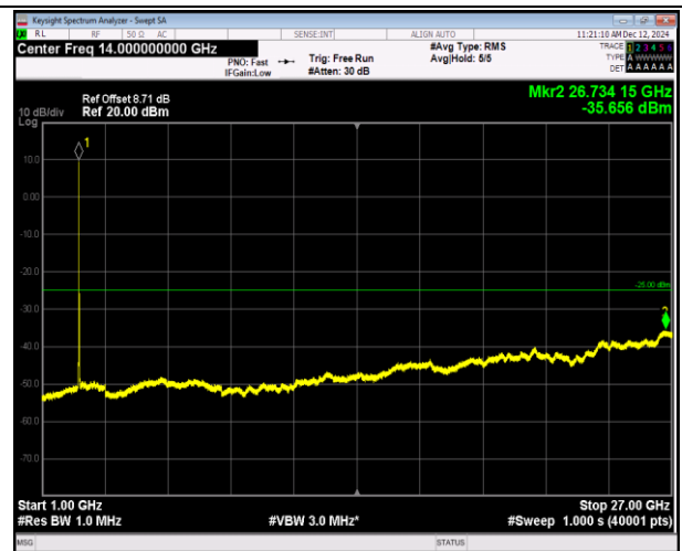
7-7-10MHz-20MHz-QPSK-QPSK-21006-21150-50RB#0-10 0RB#0-1000~27000MHz-PASS
