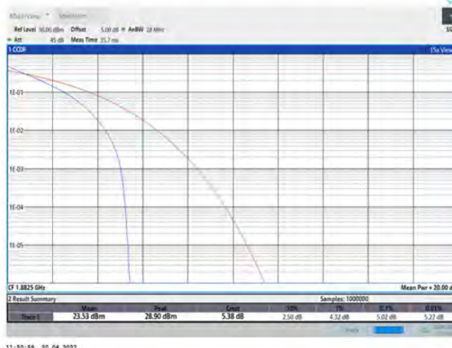
Band25-20MHz-QPSK-26365-100RB#0
