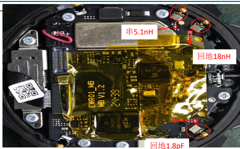
GPS L1/L5/BT匹配
