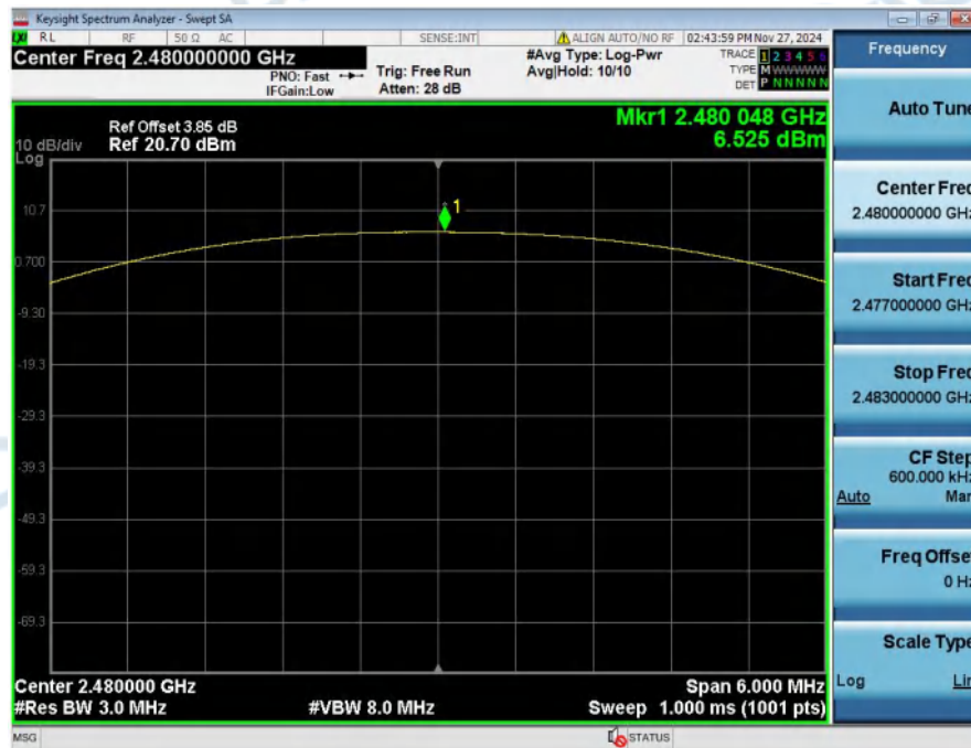
Peak_Output_Power_NVNT_ANT1_1Mbps_2480
