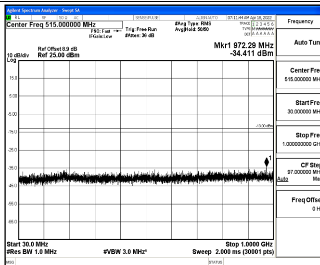
Band2-1.4MHz-QPSK-18900-1-0-Low-30-1000--34.41-PASS
