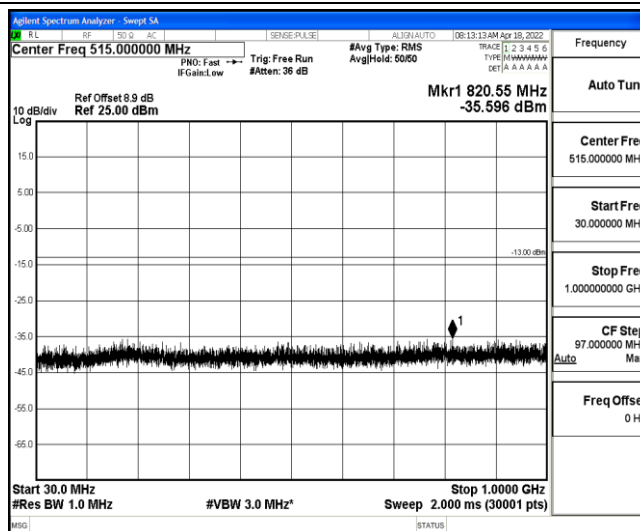
Band2-5MHz-QPSK-18900-1-0-Low-30-1000--35.6-PASS
