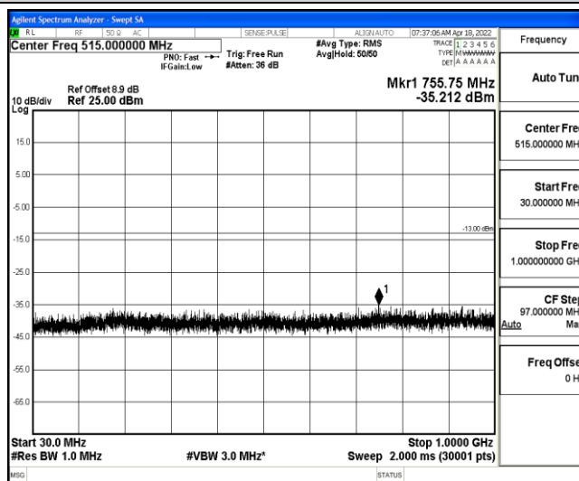
Band2-3MHz-QPSK-18615-1-0-Low-30-1000--35.21-PASS
