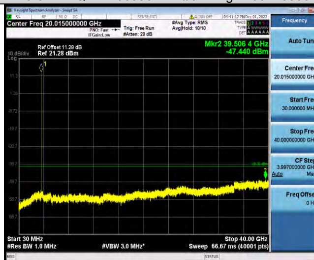
Band48-5MHz-QPSK-56715-1RB#0-Range1:30~40000MHz
