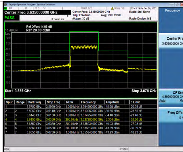
Band48-20MHz-QPSK-56640-1RB#0
