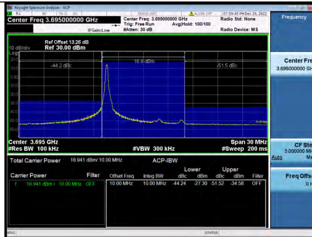
Band48-10MHz-QPSK-56690-50RB#0
