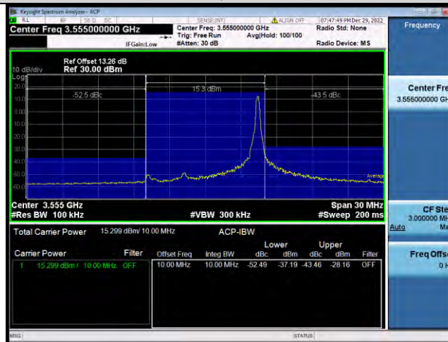
Band48-10MHz-QPSK-55290-50RB#0
