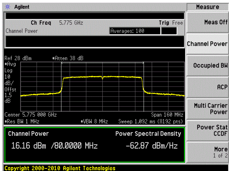
Ant-7
