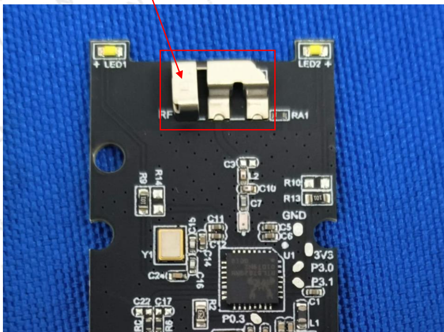
2.4G Antenna
