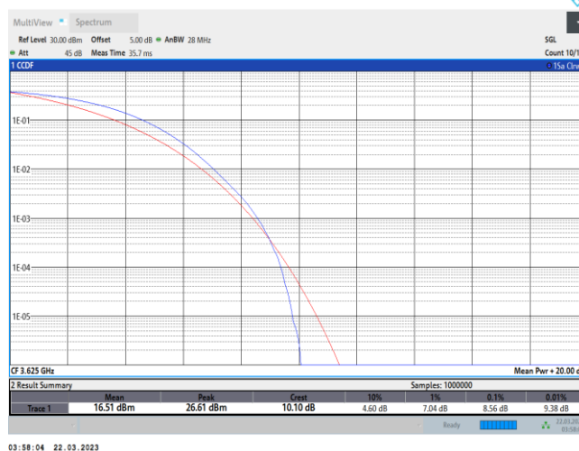
48-48-20MHz-20MHz-QPSK-QPSK-55891-56089-100RB#0-100RB#0
