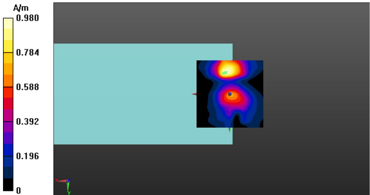
Fig A.12 T-Coil WCDMA Band 2-Y
