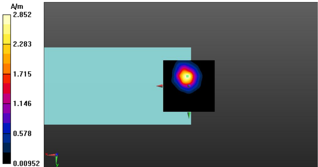
Fig A.10 T-Coil GSM 850-Z
