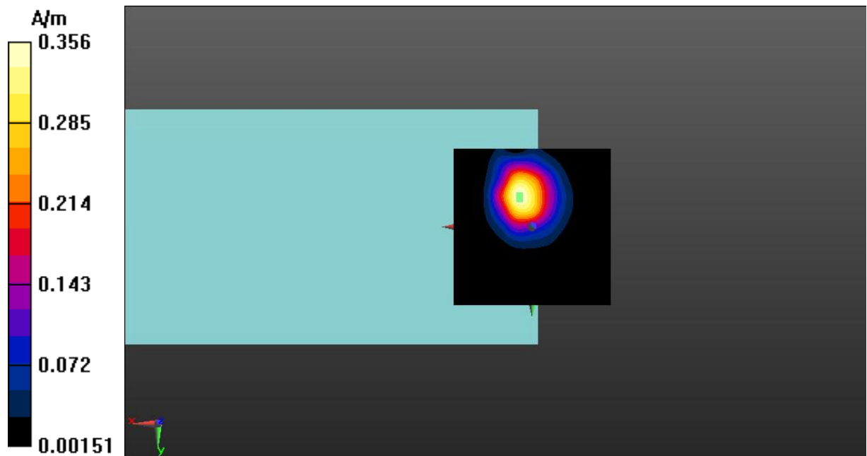
Fig A.12 T-Coil WCDMA Band 2-Z
