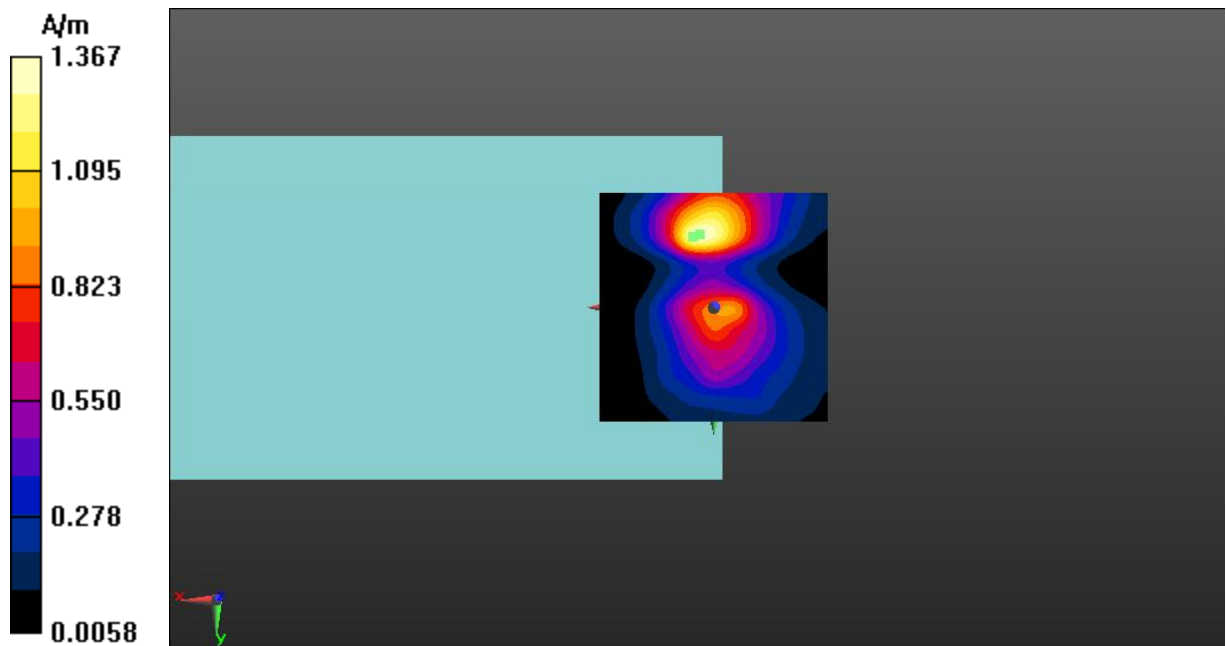
Fig A.10 T-Coil GSM 850-Y
