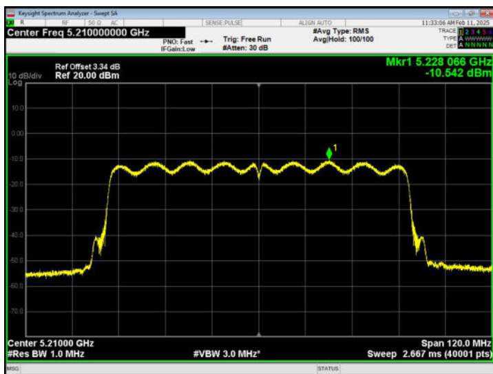
802.11ac80 - CH 42
