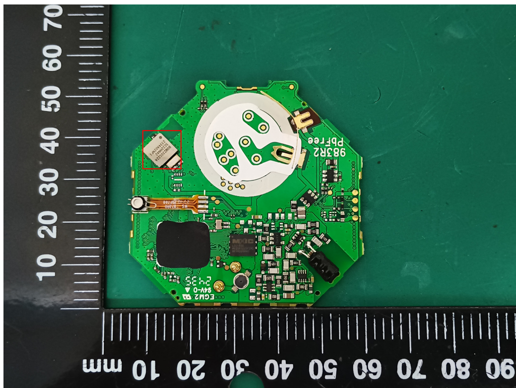
BLE ANT
