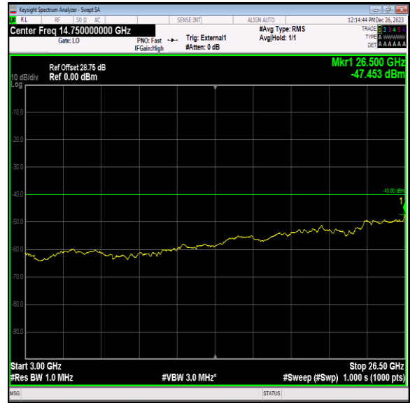
Band40_10MHz_QPSK_38750_1RB#0_3000~26500_3000~2 6500
