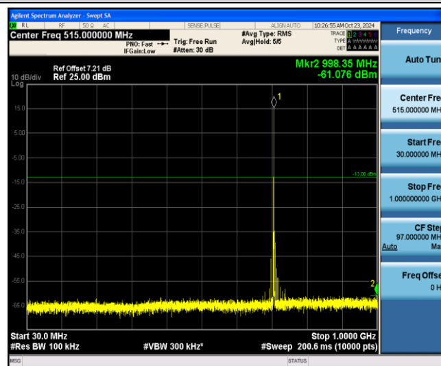
Band12-3MHz-QPSK-23165-1-0-Low-30-1000--61.08-PASS
