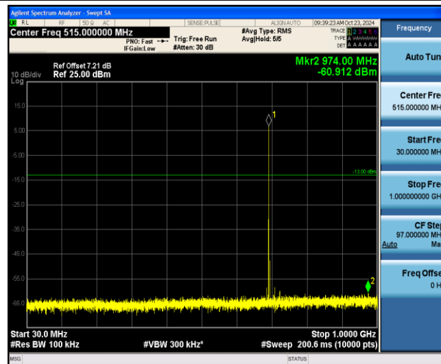
Band12-1.4MHz-16QAM-23017-1-0-Low-30-1000--60.91-PASS
