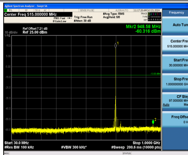
Band12-5MHz-QPSK-23095-1-0-Low-30-1000--60.32-PASS
