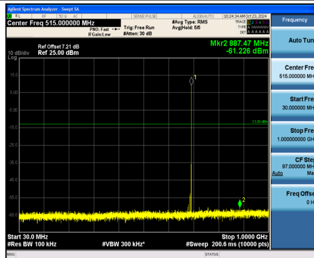
Band12-3MHz-QPSK-23025-1-0-Low-30-1000--61.23-PASS
