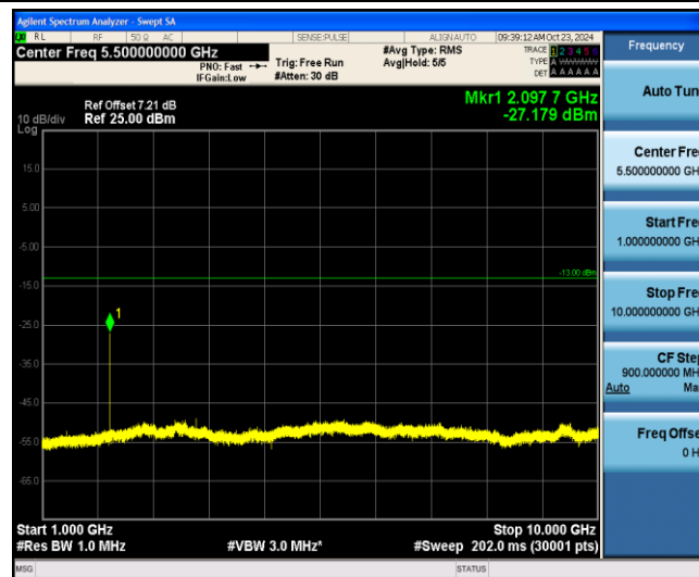
Band12-1.4MHz-QPSK-23017-1-0-Low-1000-10000--27.18-PASS
