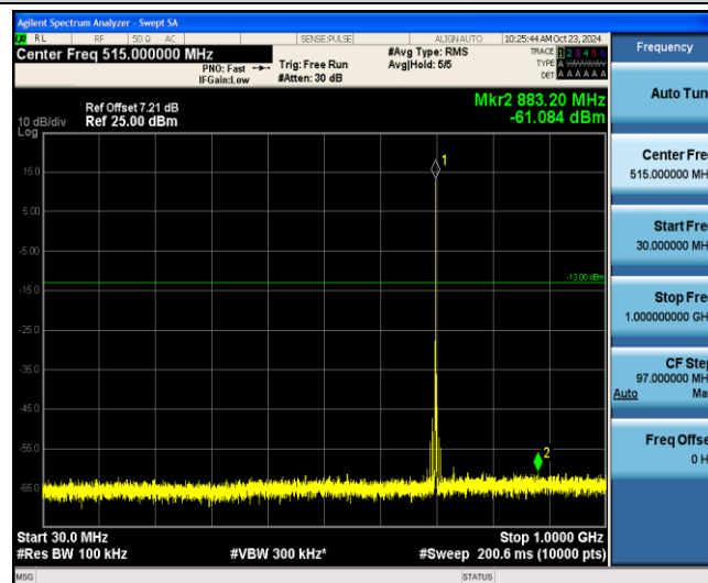
Band12-3MHz-QPSK-23095-1-0-Low-30-1000--61.08-PASS
