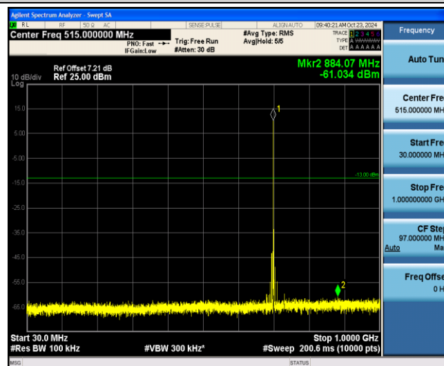
Band12-1.4MHz-QPSK-23095-1-0-Low-30-1000--61.03-PASS
