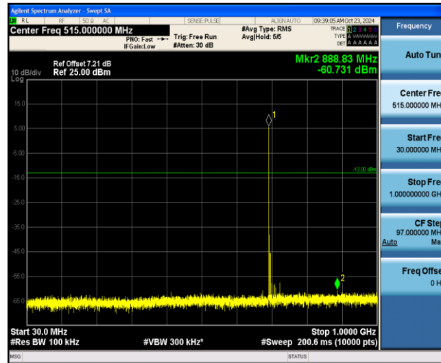
Band12-1.4MHz-QPSK-23017-1-0-Low-30-1000--60.73-PASS
