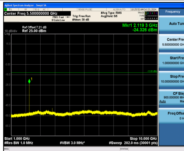
Band12-3MHz-QPSK-23095-1-0-Low-1000-10000--24.33-PASS
