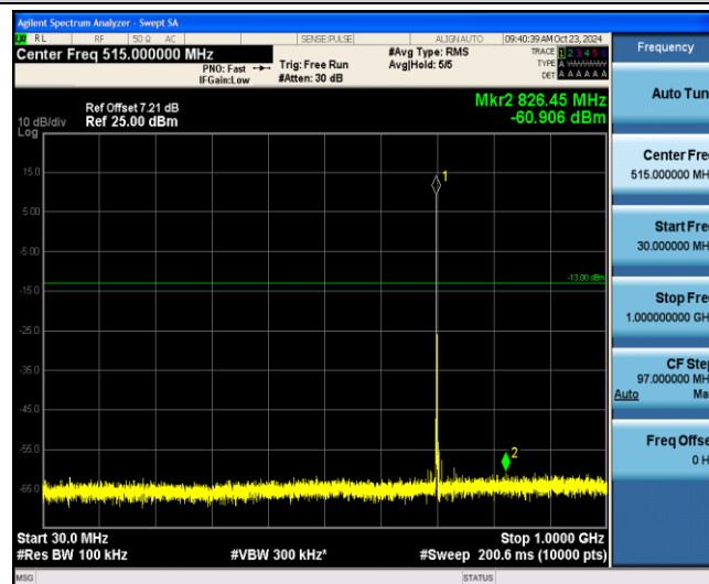
Band12-1.4MHz-16QAM-23095-1-0-Low-30-1000--60.91-PASS
