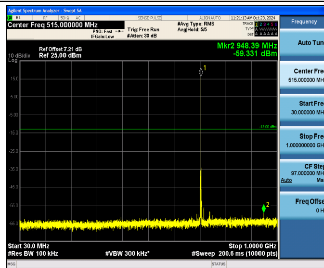
Band12-5MHz-QPSK-23155-1-0-Low-30-1000--59.33-PASS
