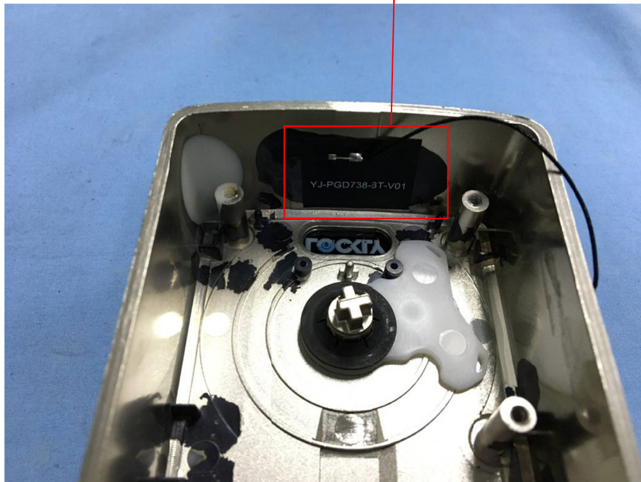
BLE Antenna
