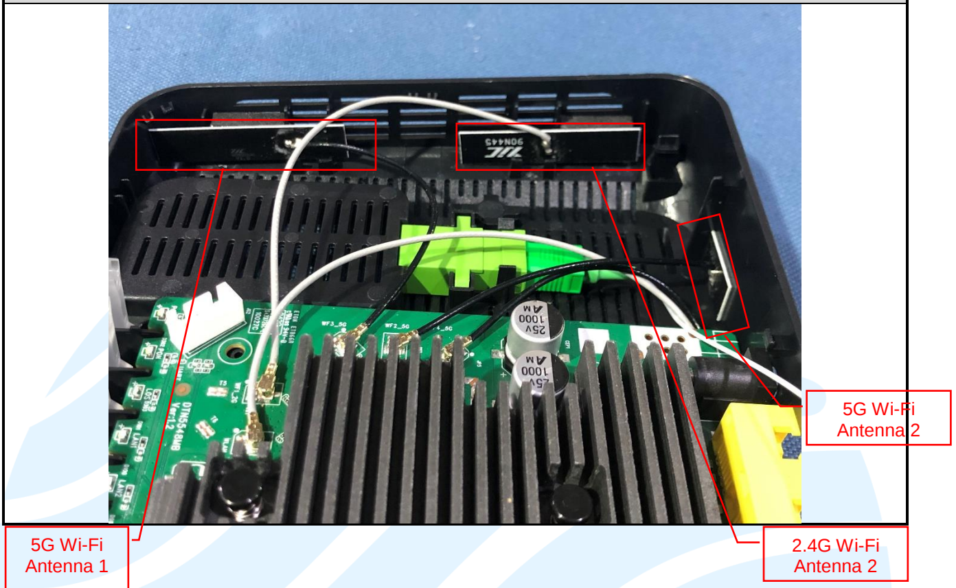
EUT Photo
