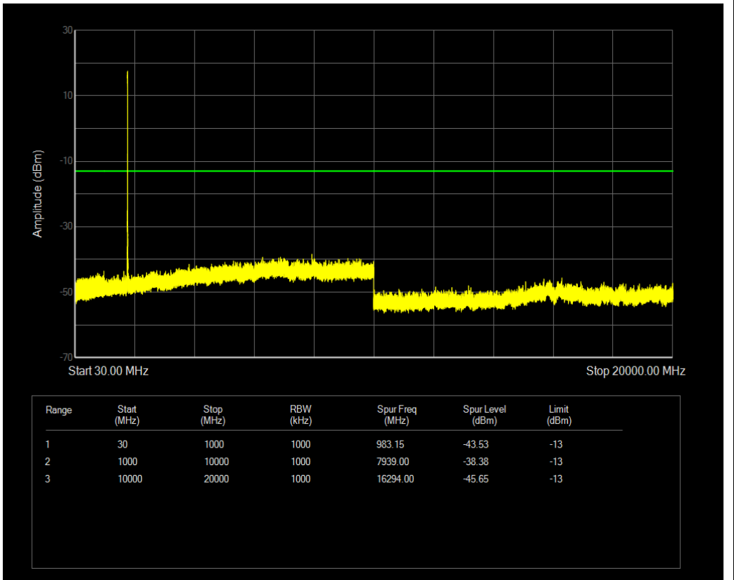
n66 SCS=15kHz DFT_BPSK BW=5MHz Channel=355500 RB=1@0
