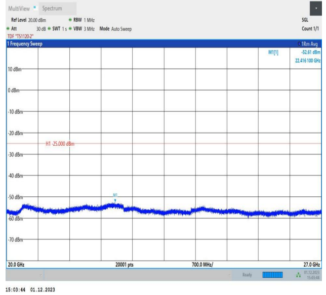
7-7-15MHz-10MHz-QPSK-QPSK-21051-21171-75RB#0-50RB #0-20000~27000MHz-PASS
