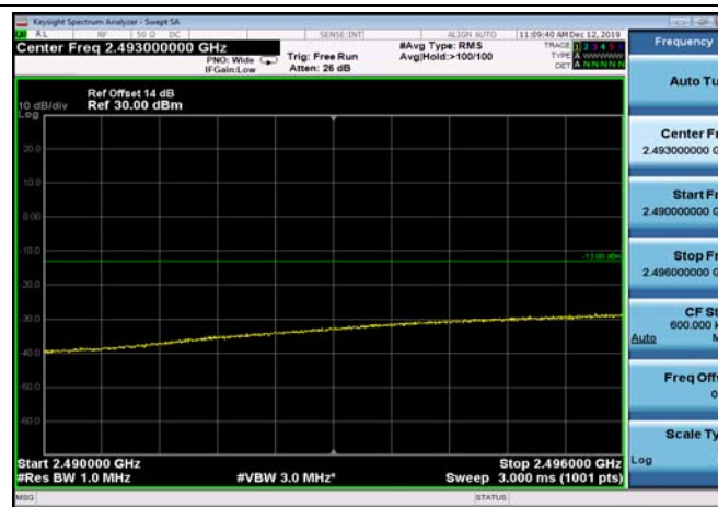
FDD07_10MHz_2505_Q16_fullRB_ExtraBand s_Range_2490~2496
