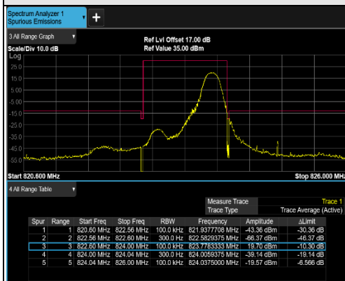
1RB#MAX (823.3MHz)
