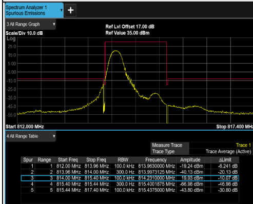
1RB#0 (814.7MHz)
