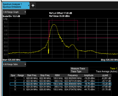
1RB#0 (823.3MHz)
