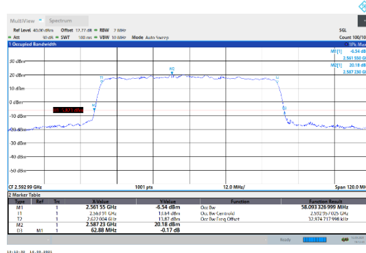
N41-30kHz-60MHz-CP-QPSK-Mid-Outer_Full---PASS
