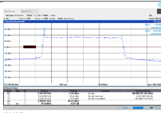
N41-30kHz-90MHz-CP-QPSK-Mid-Outer_Full---PASS
