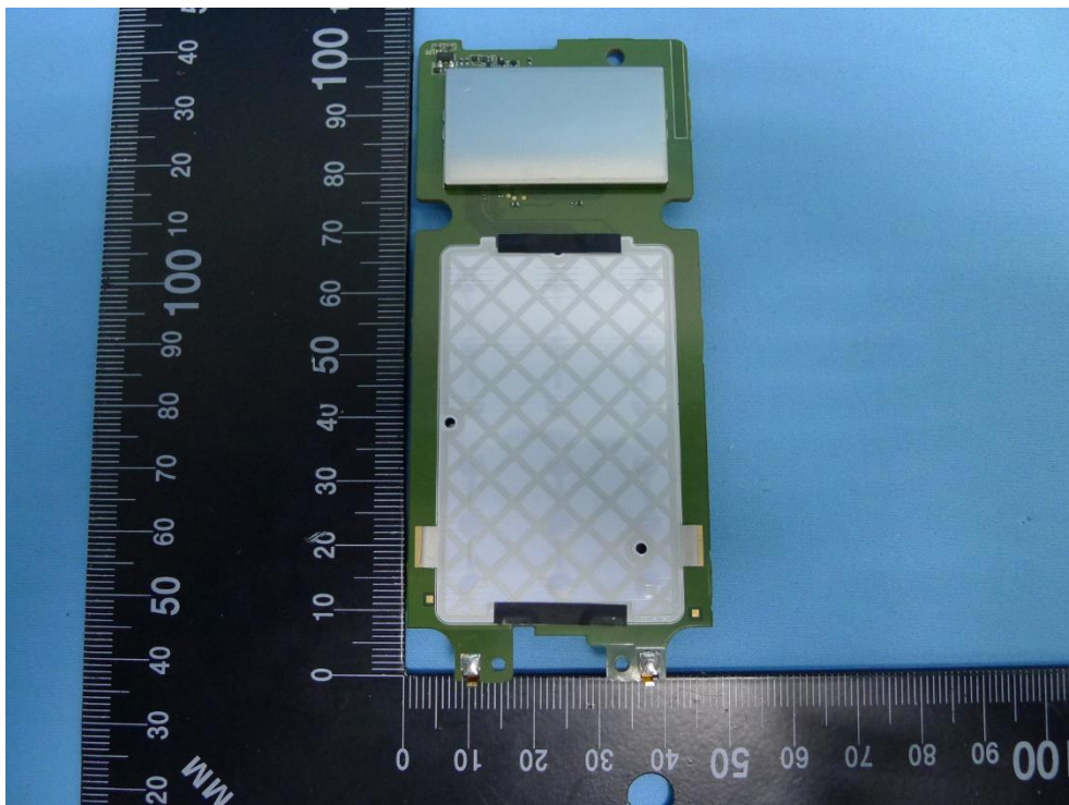
(6) EUT Photos
