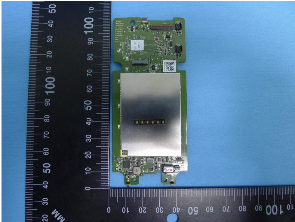
(5) EUT Photos
