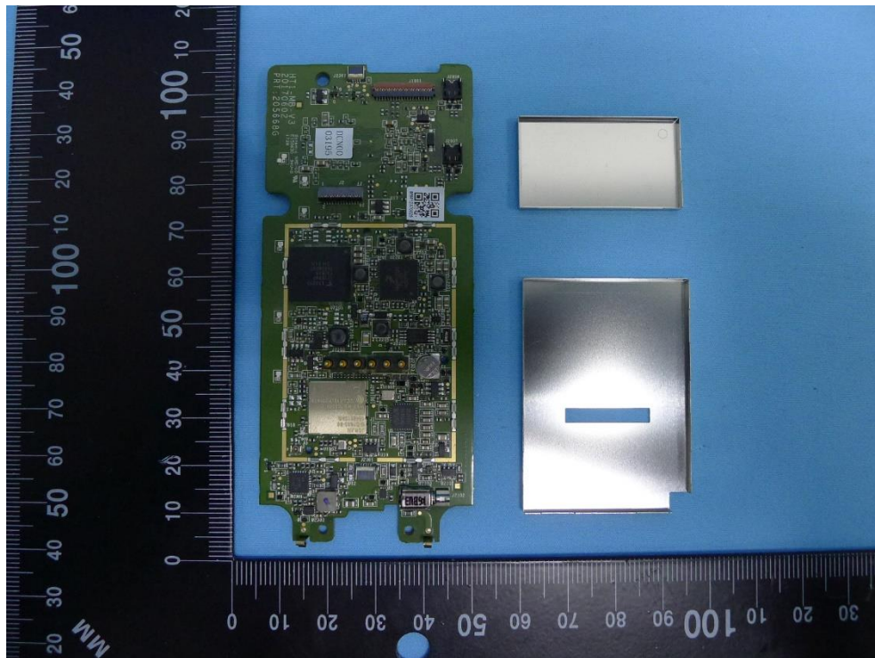
(7) EUT Photos
