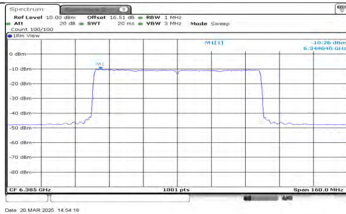
11AX80MIMO_Ant1_6385
