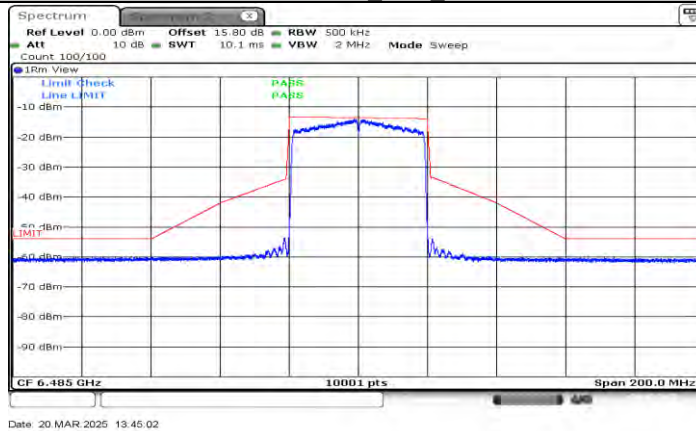
11AX40MIMO_Ant1_6485
