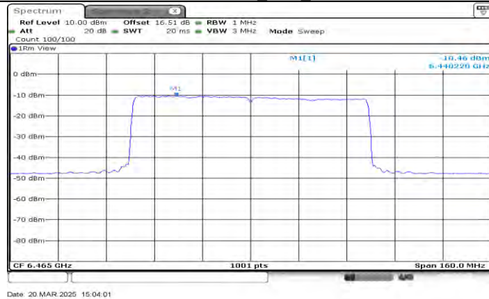
11AX80MIMO_Ant1_6465
