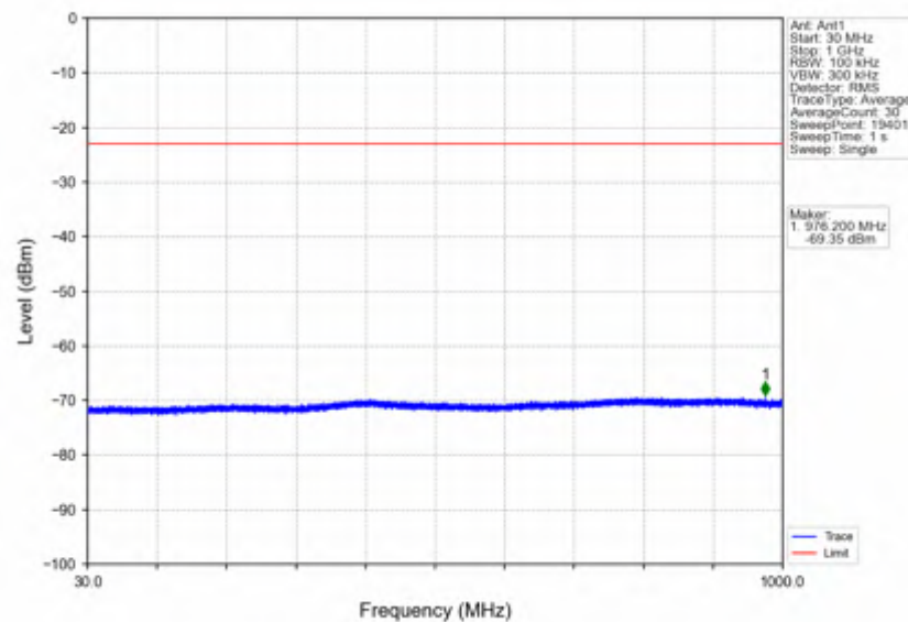
n7 15kHz SISO NTN 50MHz DFT-s-OFDM QPSK 2525MHz Edge 1RB Left
