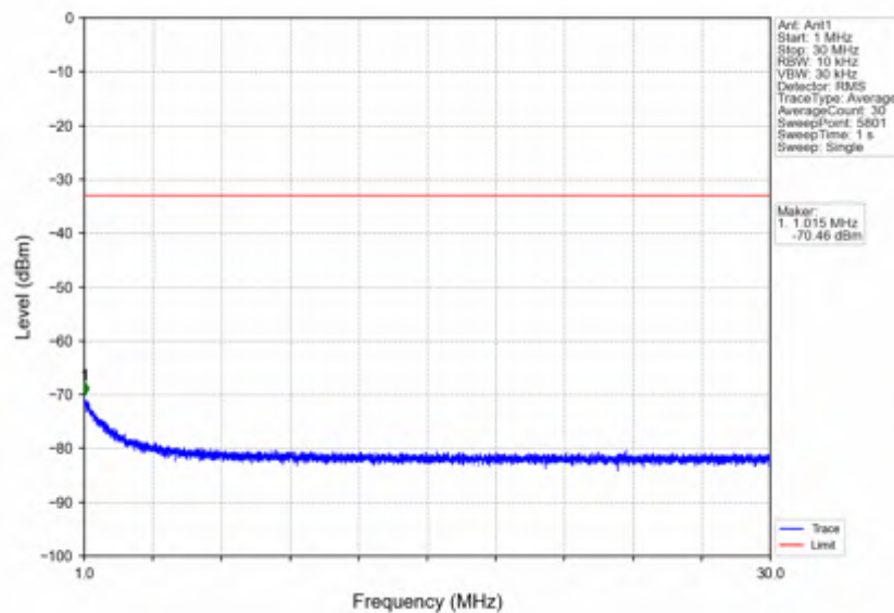
n7 15kHz SISO NTN 30MHz CP-OFDM QPSK 2535MHz Edge 1RB Left
