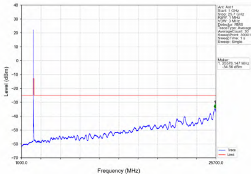
n7 15kHz SISO NTNv 30MHz DFT-s-OFDM PI/2 BPSK 2535MHz Edge 1RB Left
