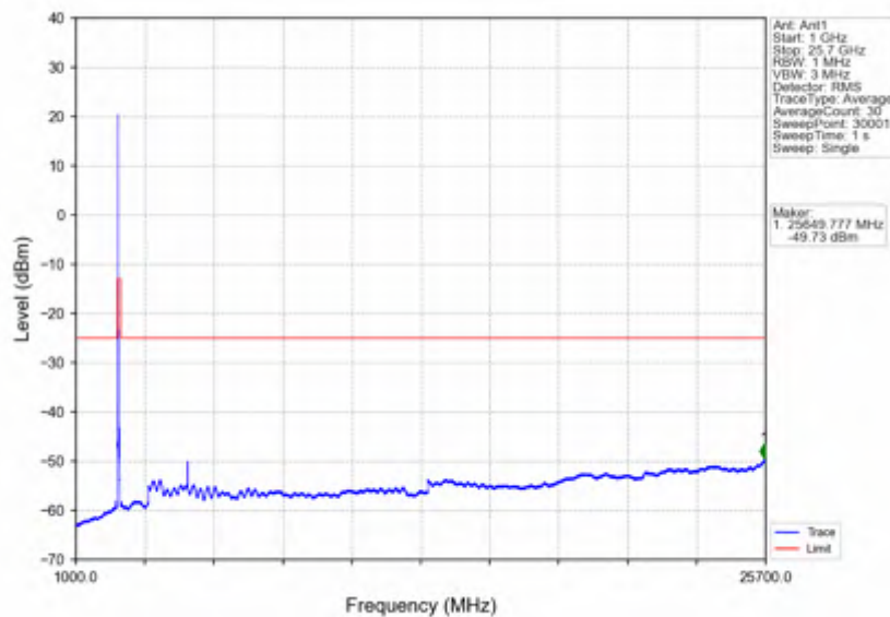
n7 15kHz SISO NTV 25MHz CP-OFDM QPSK 2535MHz Edge 1RB Left
