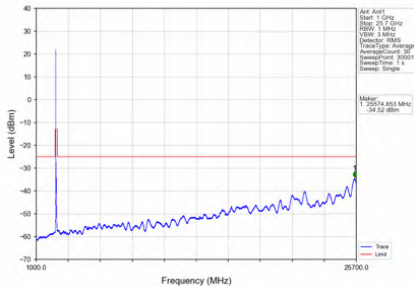
n7 15kHz SISO NTN 50MHz DFT-s-OFDM QPSK 2525MHz Edge 1RB Left
