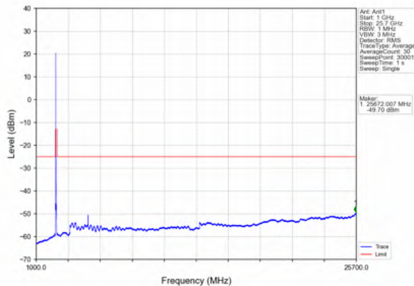
n7 15kHz SISO NTN 30MHz DFT-s-OFDM QPSK 2515MHz Edge 1RB Left
