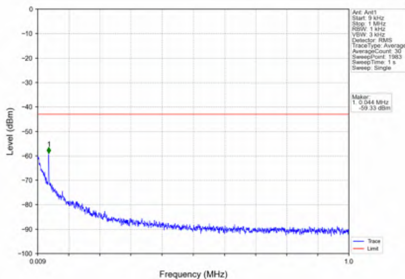
n7_15kHz_SISO_NTNV_40MHz_DFT-s-OFDM_PI/2_BPSK_2520MHz_Edge_1RB_Left
