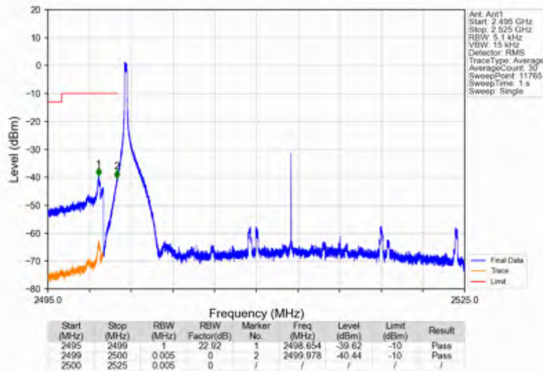
n7 15kHz SISO NTNv 25MHz CP-OFDM QPSK 2512.5MHz Edge 1RB Left
