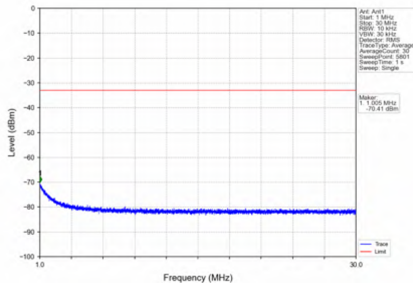
n7 15kHz SISO NTNV 40MHz DFT-s-OFDM QPSK 2520MHz Edge 1RB Left
