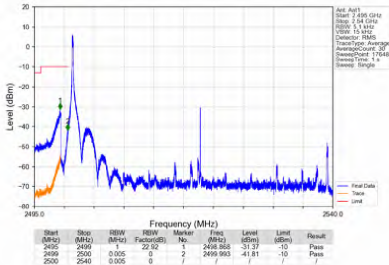
n7_15kHz_SISO_NTNV_40MHz_DFT-s-OFDM_QPSK_2520MHz_Inner_1RB_Left
