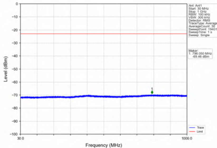
n7_15kHz_SISO_NTNV_40MHz_CP-OFDM_QPSK_2520MHz_Inner_1RB_Left
