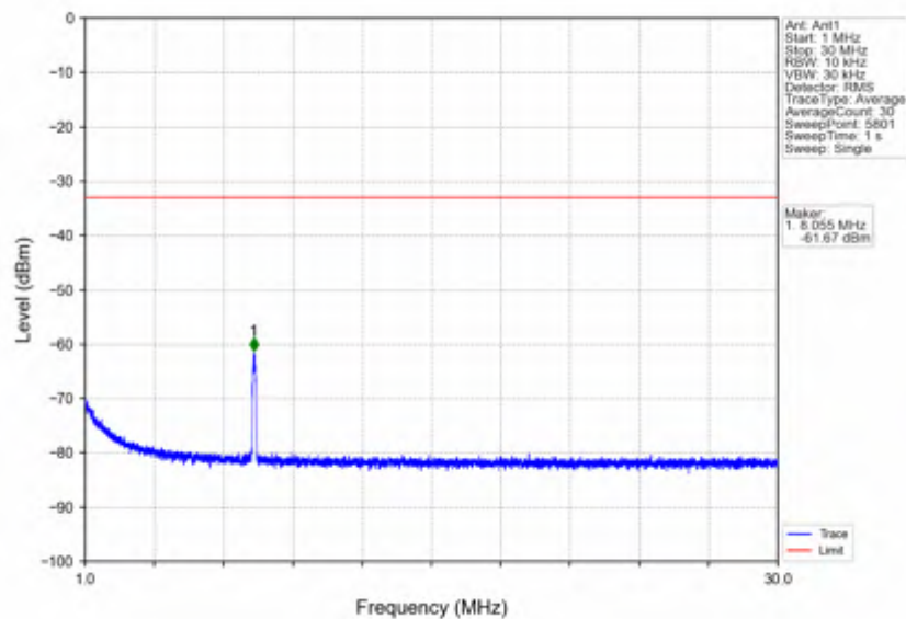
n7 15kHz SISO NTN 40MHz DFT-s-OFDM QPSK 2550MHz Edge 1RB Right
