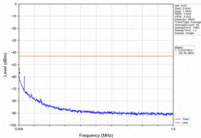
n7_15kHz_SISO_NTNV_40MHz_DFT-s-OFDM QPSK_2520MHz_Inner_1RB_Left
