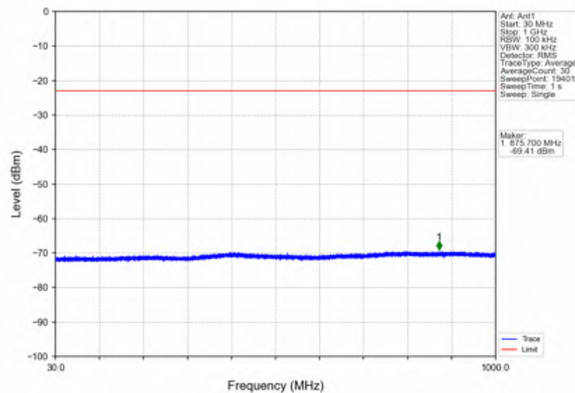
n7 15kHz SISO NTN 40MHz DFT-s-OFDM QPSK 2520MHz Edge 1RB Left
