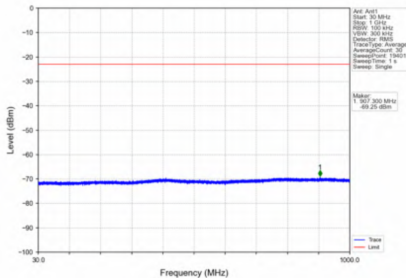
n7 15kHz SISO NTNv 30MHz DFT-s-OFDM PI/2 BPSK 2535MHz Edge 1RB Left
