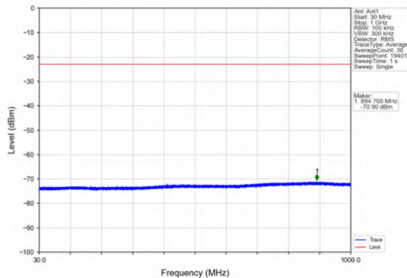
n7 15kHz SISO NTN 30MHz DFT-s-OFDM QPSK 2515MHz Edge 1RB Left
