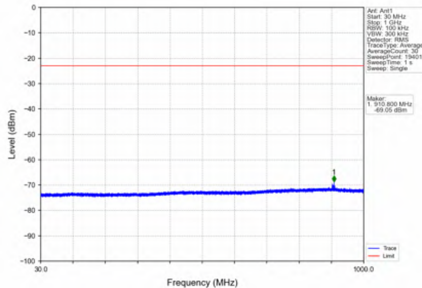
n7_15kHz_SISO_NTNV_30MHz_DFT-s-OFDM PI/2 BPSK_2515MHz_Inner_1RB_Left
