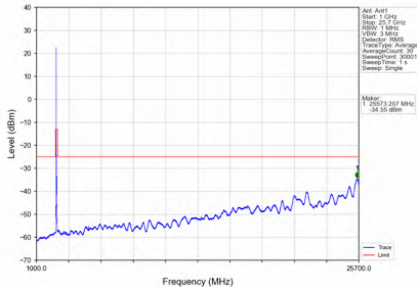
n7_15kHz_SISO_NTNV_40MHz_DFT-s-OFDM_QPSK_2520MHz_Inner_1RB_Left
