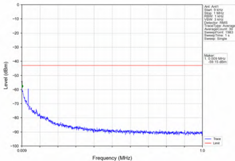
n7 15kHz SISO NTNV 40MHz DFT-s-OFDM QPSK 2535MHz Edge 1RB Left
