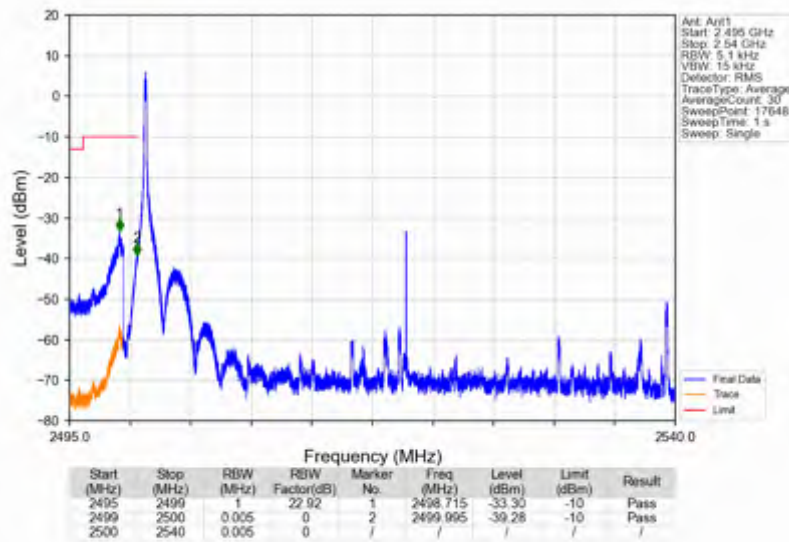
n7 15kHz SISO NTNv 40MHz DFT-s-OFDM PI/2 BPSK 2520MHz Edge 1RB Left
