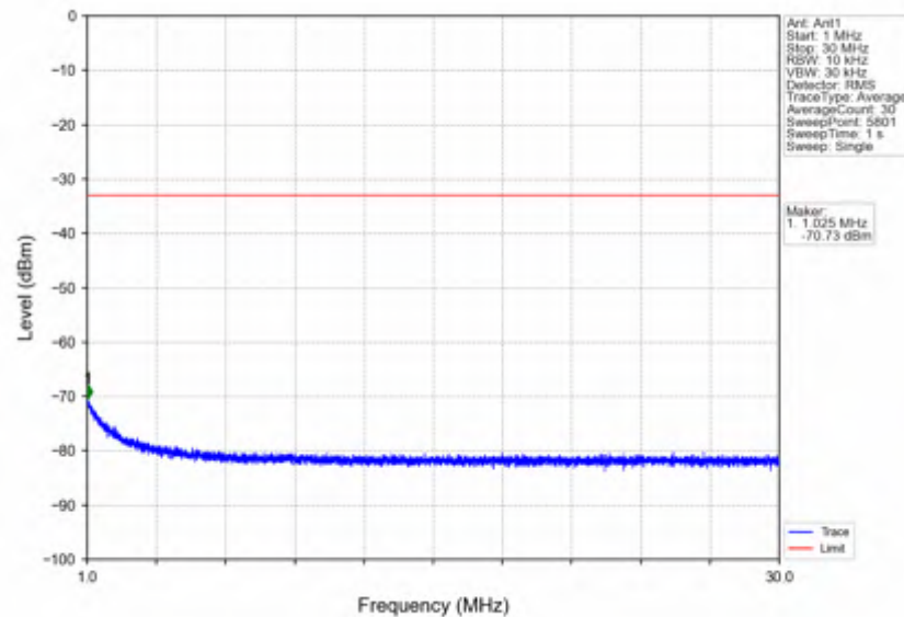
n7_15kHz_SISO_NTNV_50MHz_DFT-s-OFDM PI/2 BPSK_2525MHz_Inner_1RB_Left
