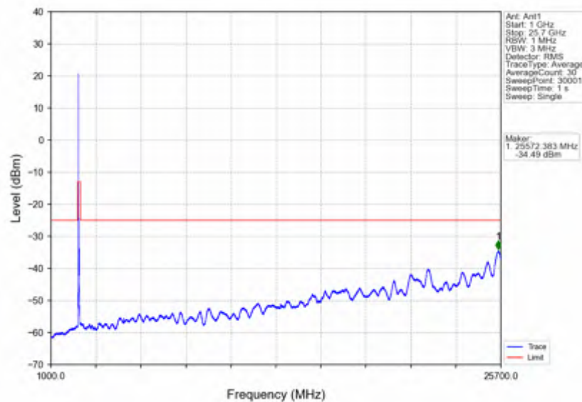
n7 15kHz SISO NTN 40MHz DFT-s-OFDM QPSK 2520MHz Edge 1RB Left
