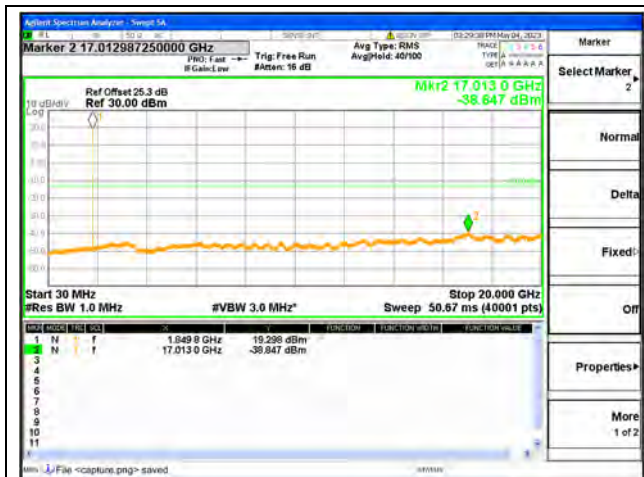
Band2 / 1.4MHz / Low CH / QPSK
