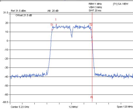
LAA-2 carriers(CA_46A-46A) / Chain 0 : CH48
