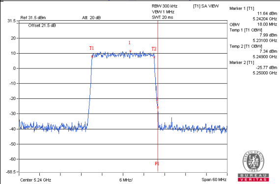
LAA-2 carriers(CA_46A-46A) / Chain 1 : CH48
